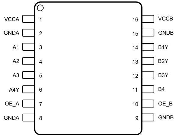
图 4-5. TXG1041-Q1 DBQ 16 引脚 QSOP 顶视图
