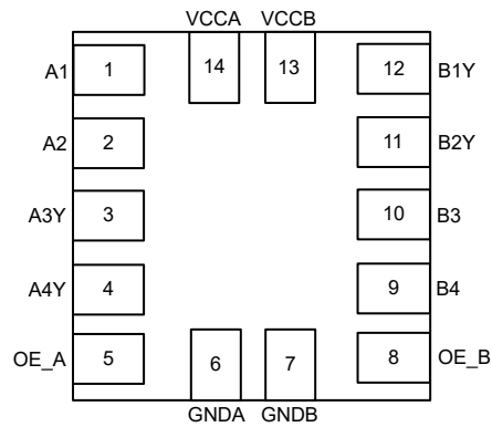
图 4-2. TXG1042-Q1 RUC 封装 14 引脚 X2QFN 顶视图
