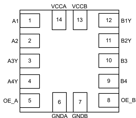
图 4-2. TXGx042RUC 封装 14 引脚 X2QFN 顶视图
