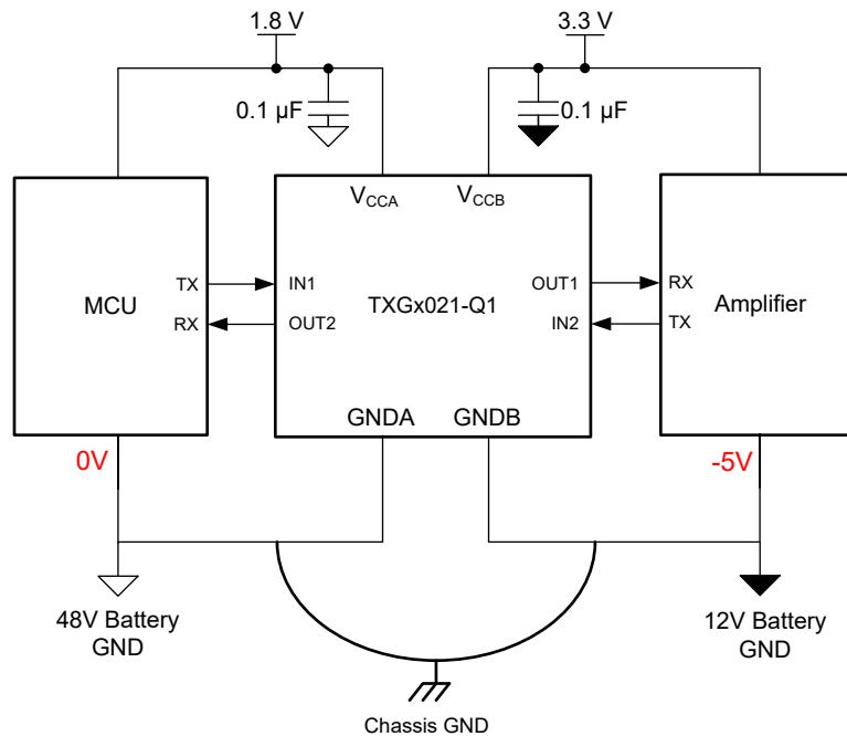
图 8-1. 汽车中的 TXG1021-Q1
