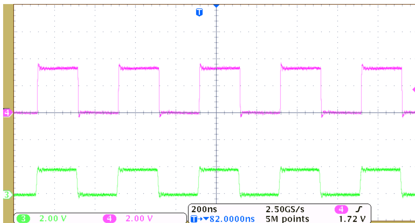
图 8-2. 2.5MHz 信号的电平转换
