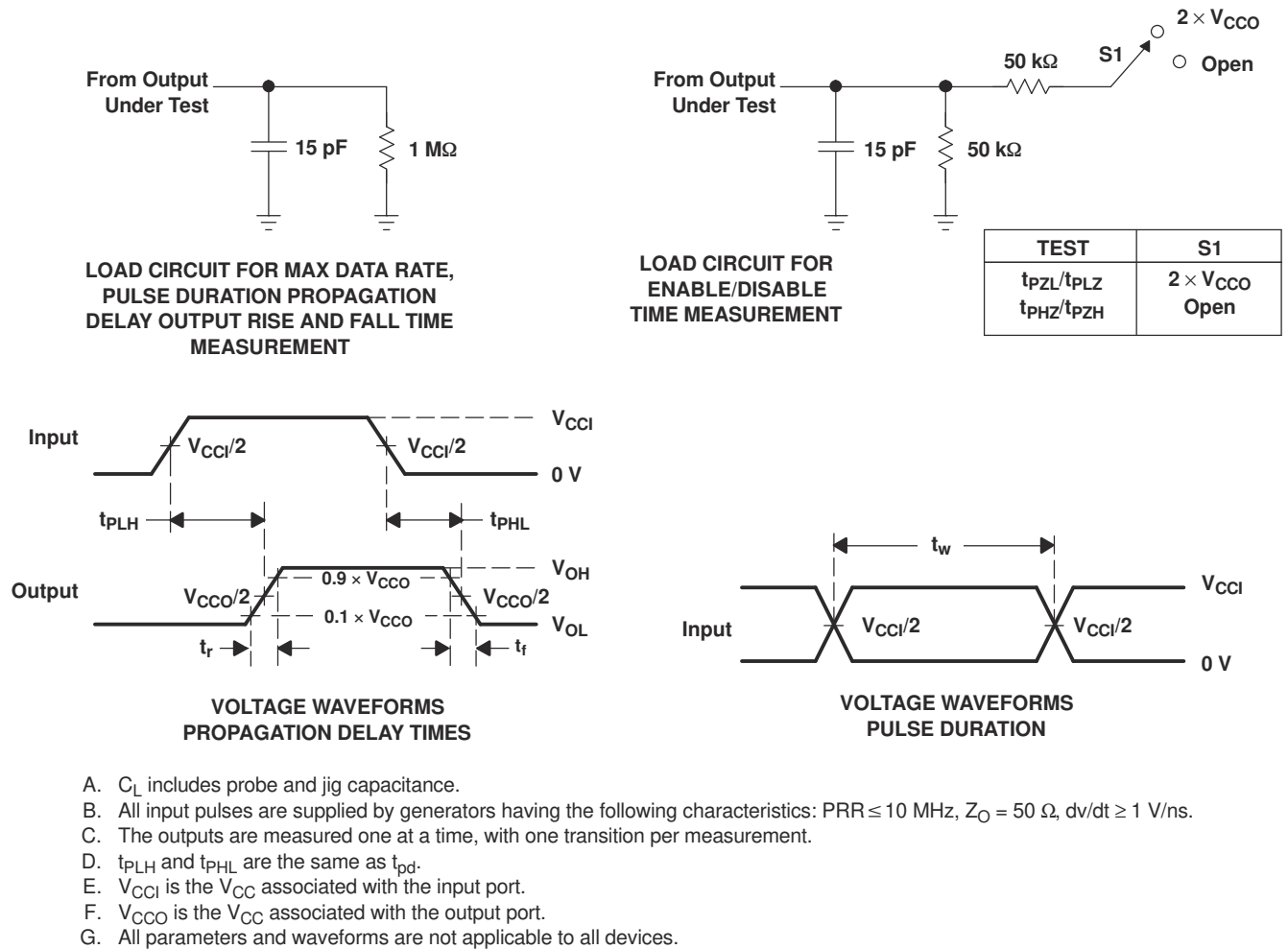
图 6-1. 负载电路和电压波形
