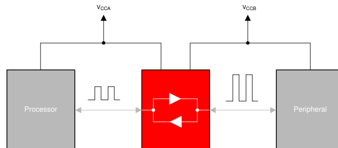
TXB0108-Q1 典型应用方框图
