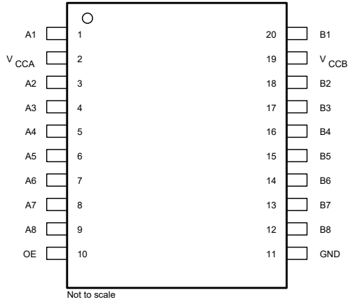
图 4-1. PW 封装 ( 顶视图 )
