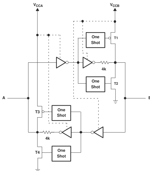
图 7-1. TXB0108-Q1 I/O 单元架构
