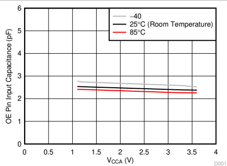
图 5-1. OE 引脚的输入电容 (C i ) 与电源 (V CCA )
