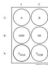
图 5-4. YZP Package, 6-Ball DSBGA (Bottom View)
