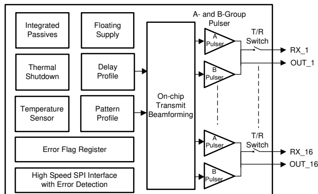
简化方框图
