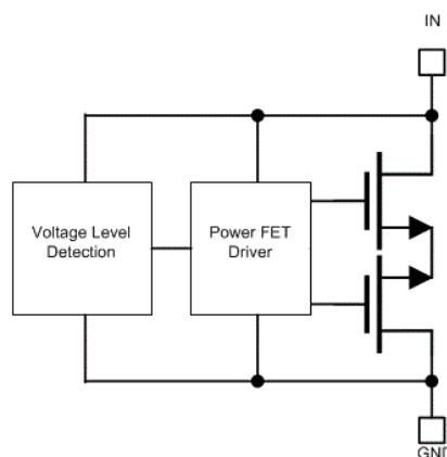
功能方框图
