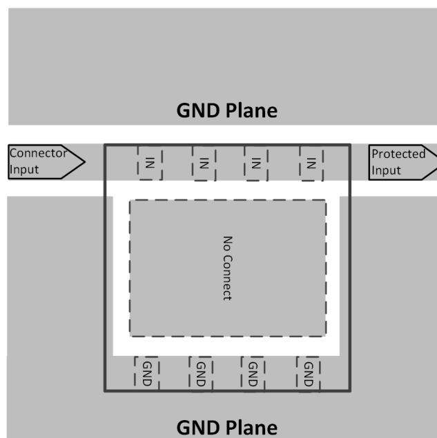
图 10. TVS2701 Layout
