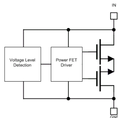
功能方框图
