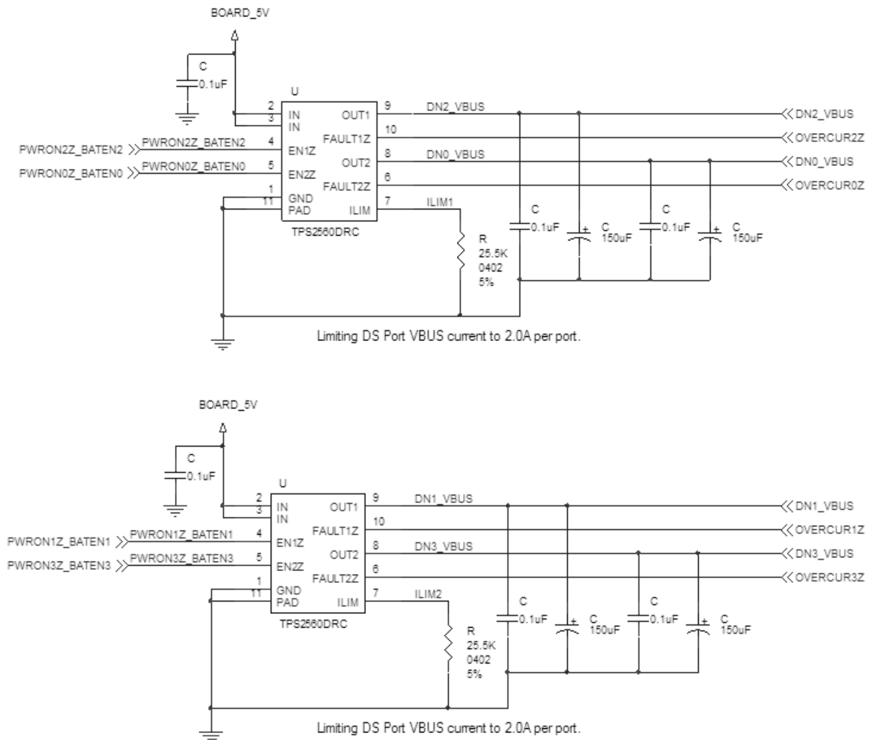
图 8-7. VBUS Power Switch Implementation
