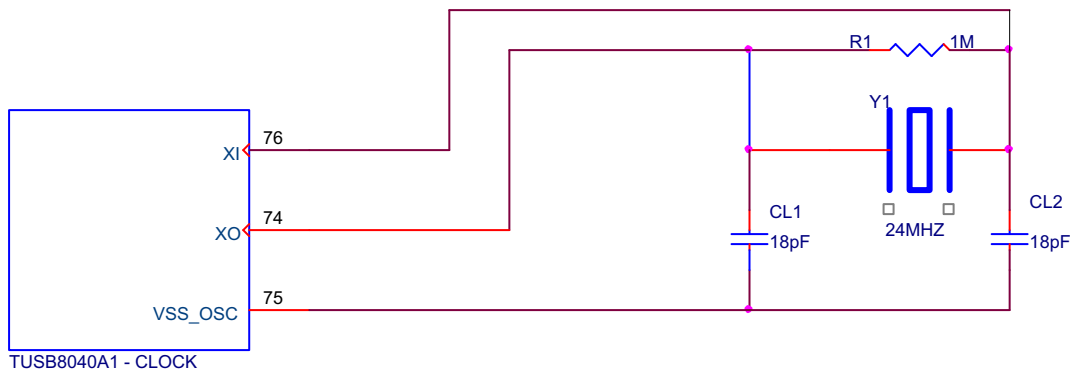
图 6-1. TUSB8040A1 Clock
