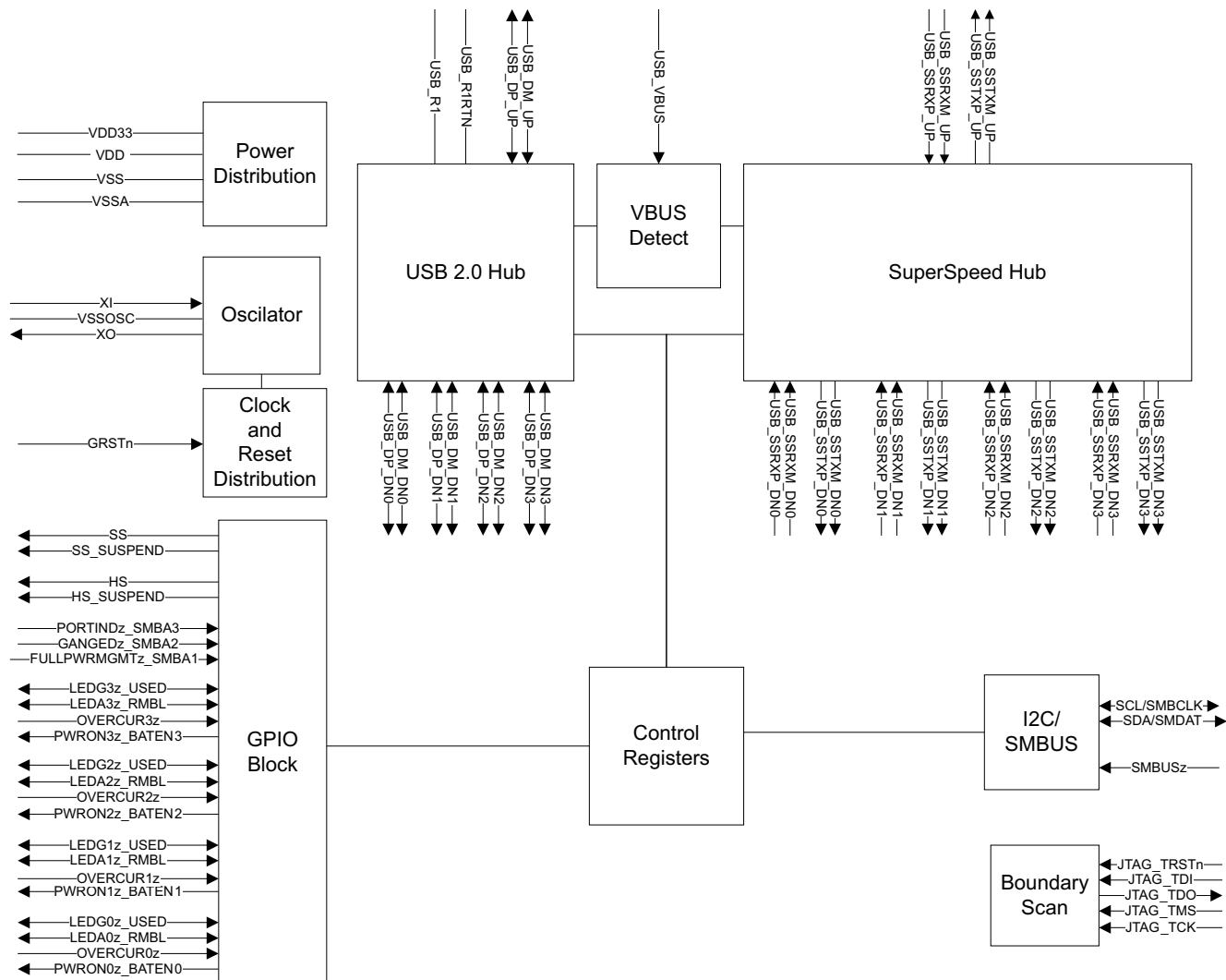
功能方框图
