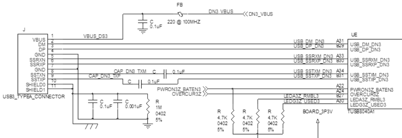
图 8-6. Downstream Port 4 Implementation
