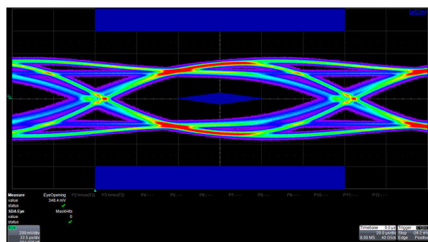
图 8-14. Downstream Port 4
