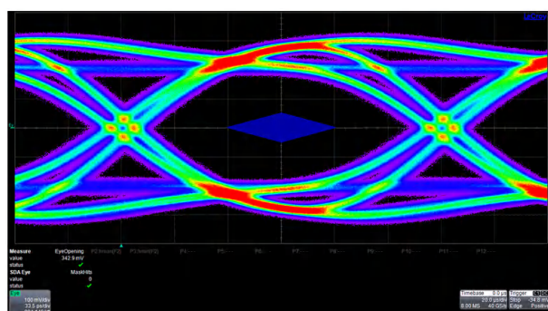
图 8-12. Downstream Port 2
