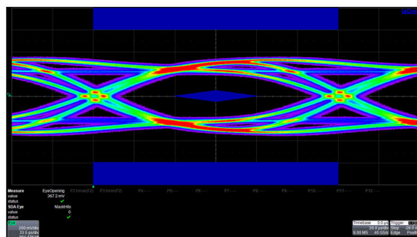
图 8-11. Downstream Port 1
