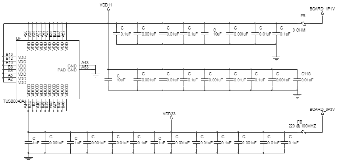
图 8-9. Power Implementation
