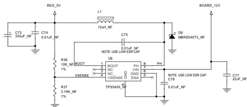
图 7-7. Reference Design 5
