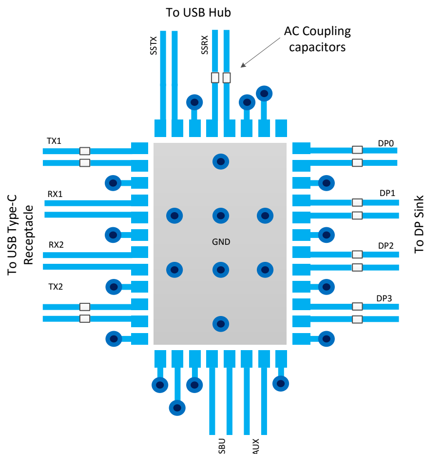
图 11-1. Layout Example
