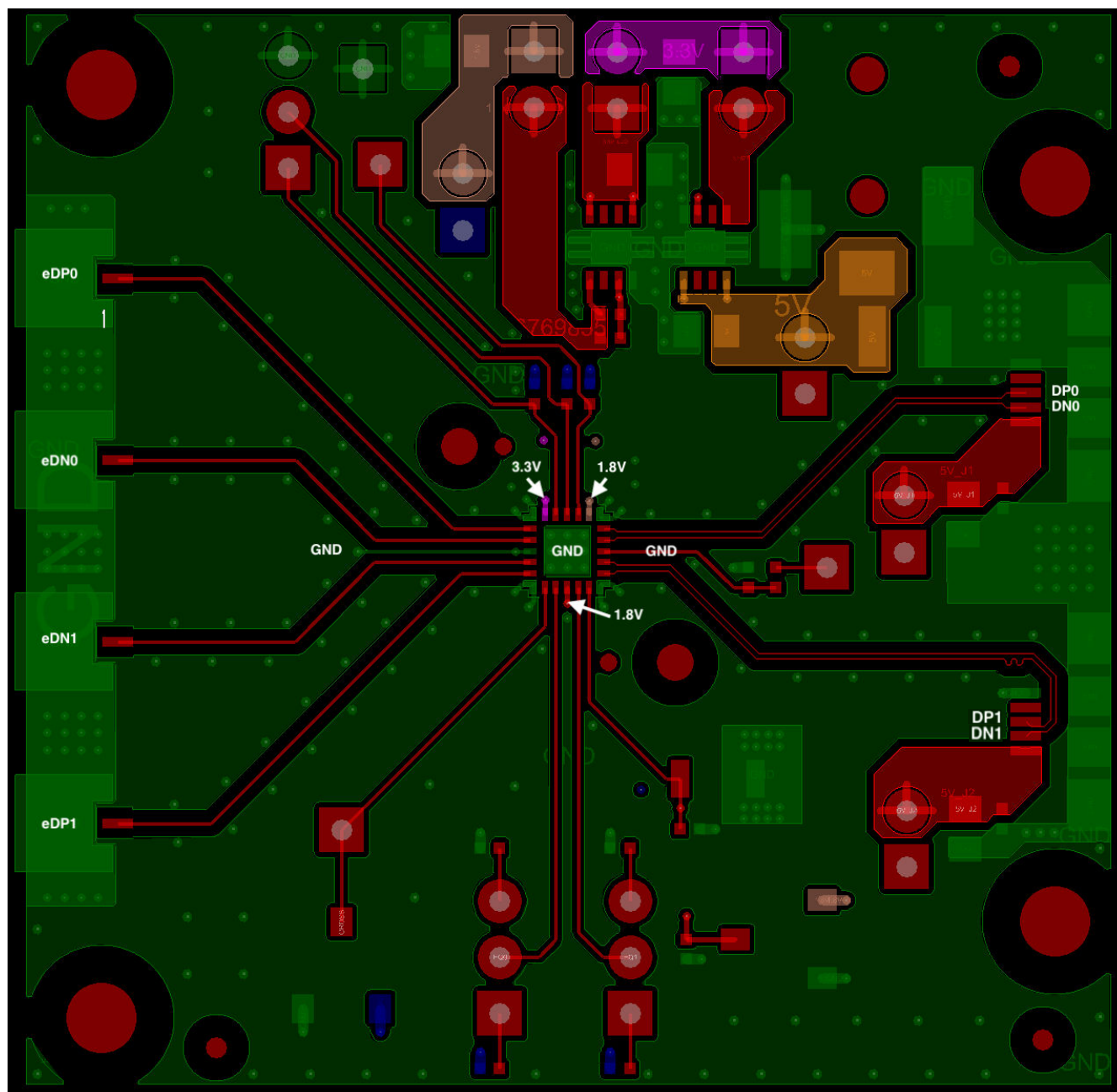
图 8-5. VQFN Example Layout
