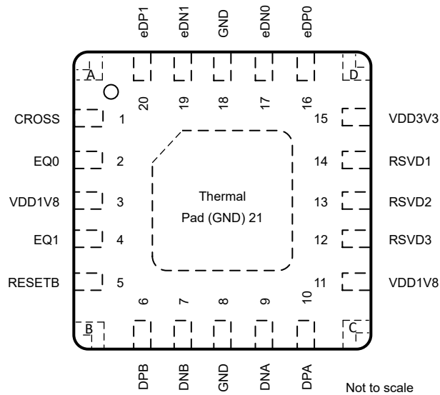
图 4-2. 0.5-mm Pitch RZA Package, 20-Pin VQFN (Top View)
