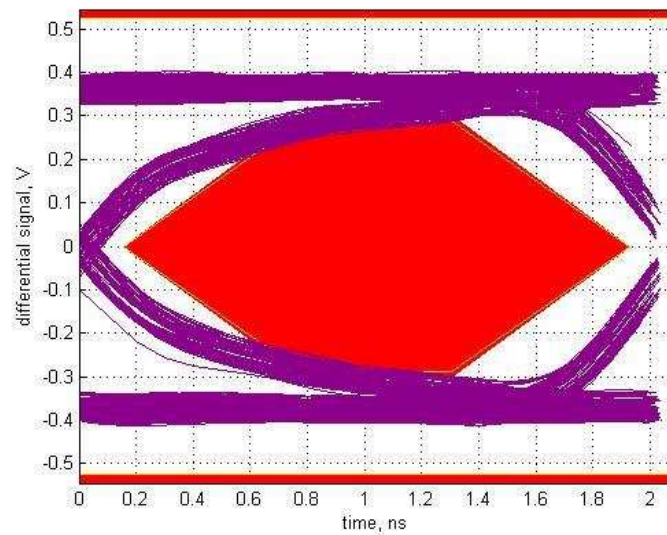
图 9. No TUSB215
