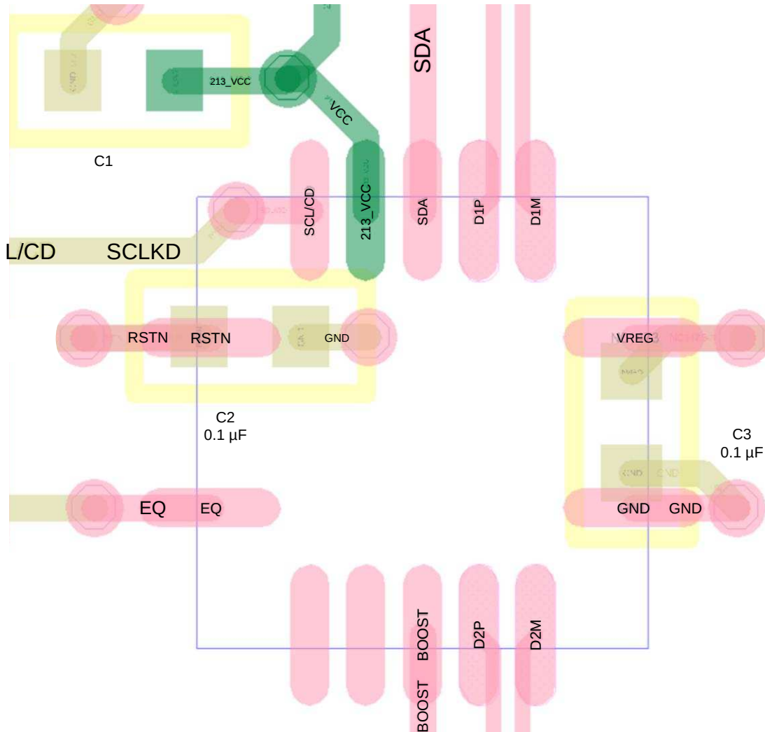
图 22. Layout Example
