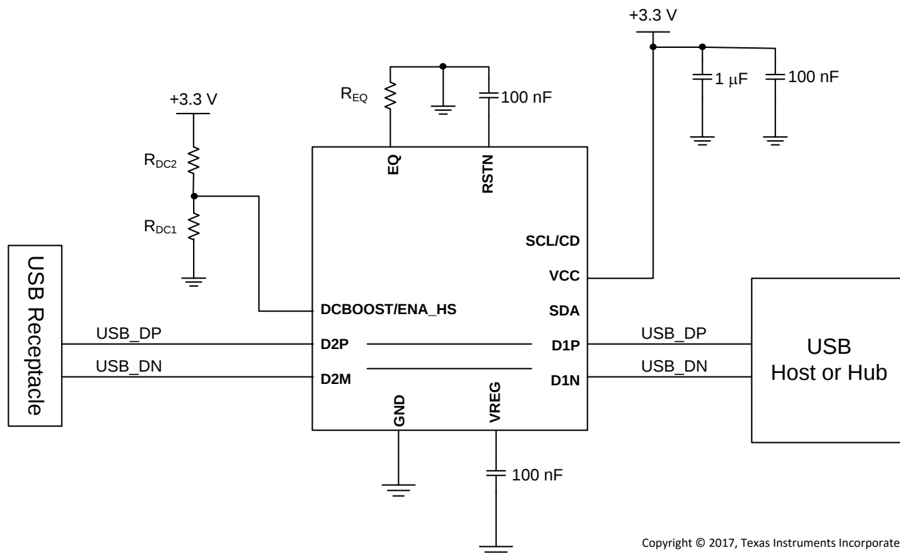
图 7. Reference Schematic
