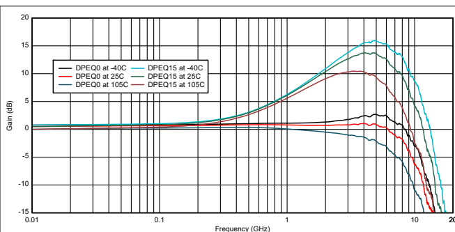
图 5-2. 不同温度下的 DisplayPort EQ DPEQ0 和 DPEQ15
