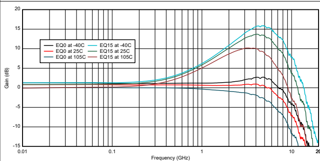
图 5-4. 不同温度下的 USB3 RX1 EQ0 和 EQ15
