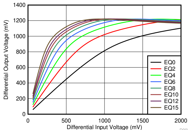
图 5-8. 5GHz 时的 USB TX (DFP) 线性曲线
