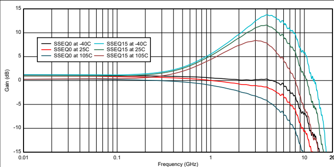
图 5-6. 不同温度下的 USB3 SSTX SSEQ0 和 SSEQ15
