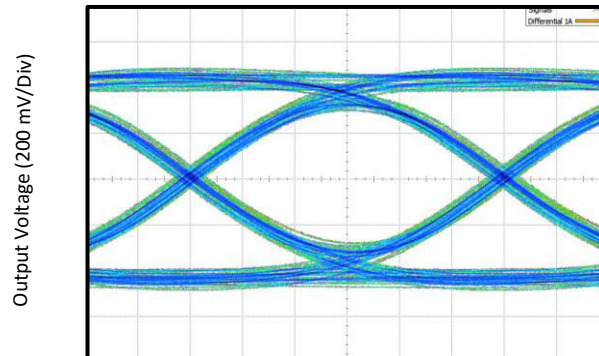
图 5-14. 在 10Gbps 时, 具有 12 英寸输入 PCB 布线的 USB 3.1 第 2 代眼图性能
