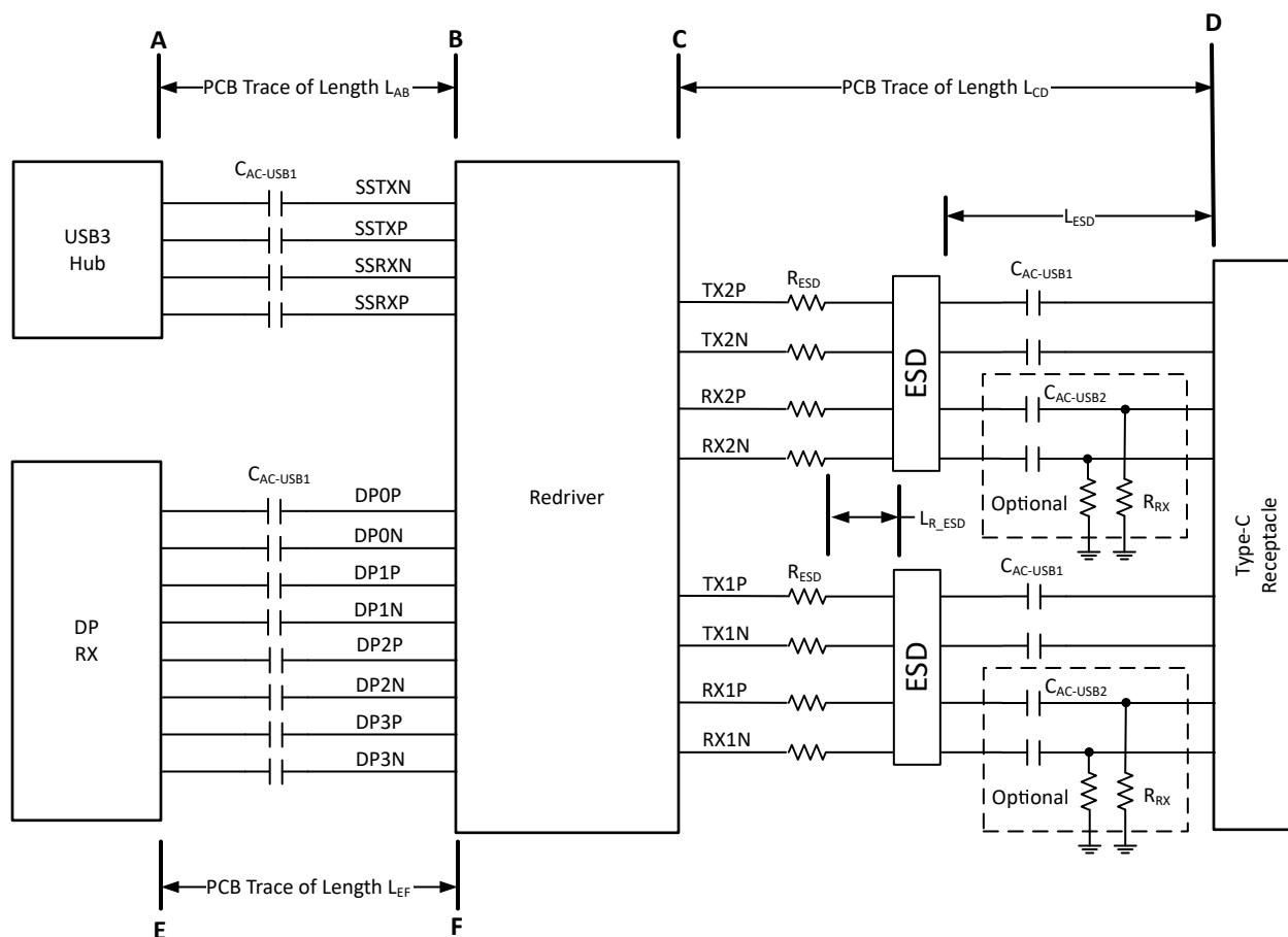
图 8-1. DP 交替模式接收端应用中的 TUSB1064-Q1
