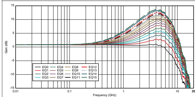
图 5-3. USB3 RX1 EQ 设置曲线
