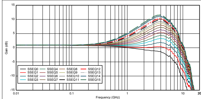
图 5-5. USB3 SSTX EQ 设置曲线
