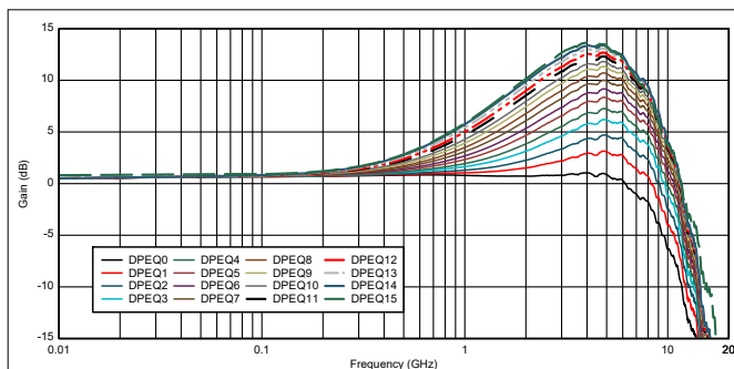
图 5-1. DisplayPort EQ 设置曲线
