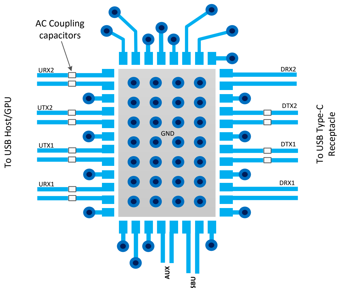
图 7-18. Example Layout
