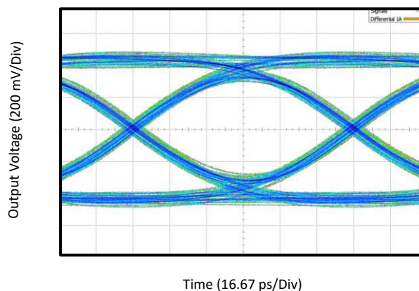
图 5-9. 在 10Gbps 时，具有 12 英寸输入 PCB 布线的 USB 3.2 第 2 代眼图性能
