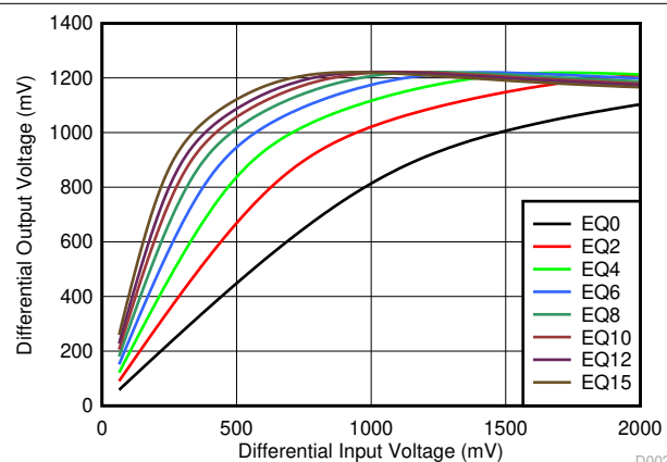
图 5-5. 5GHz 时的 USB SSTX 线性曲线
