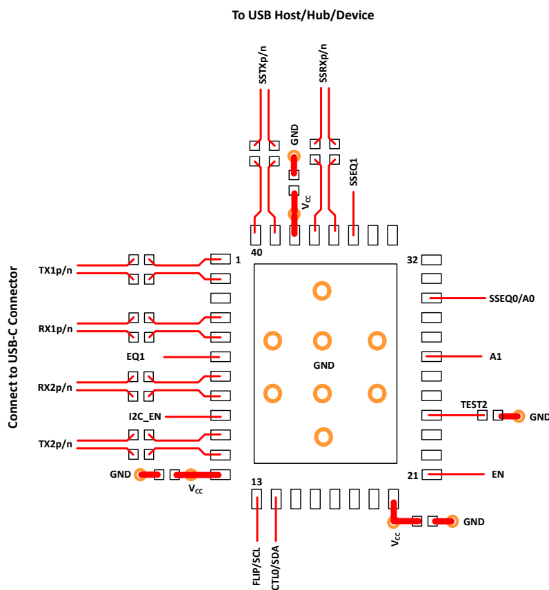
图 8-4. 布局示例
