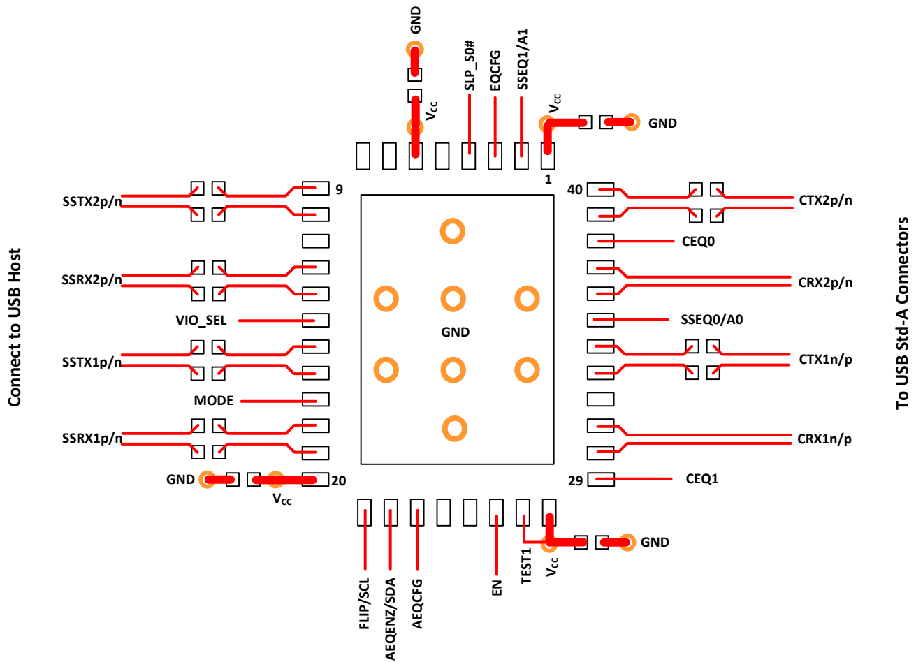
图 7-5. Layout Example
