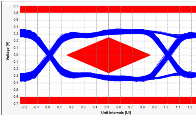
图 7-7. PCIe Gen1 TX Eye Diagram
