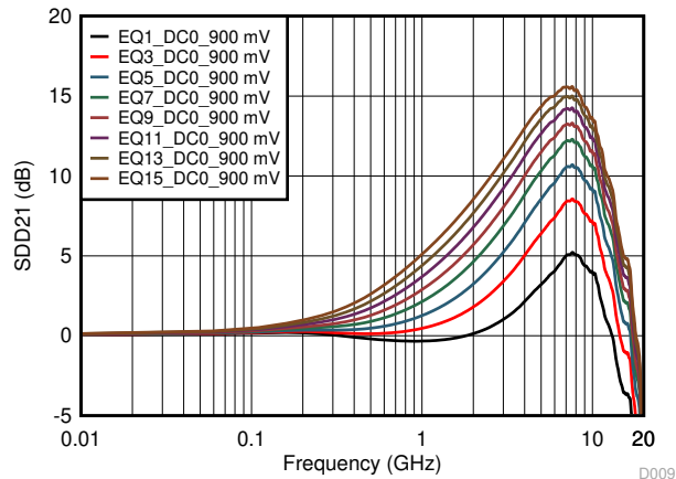
图 5-9. 900mV DC0 Gain Odd EQ Settings Curves
