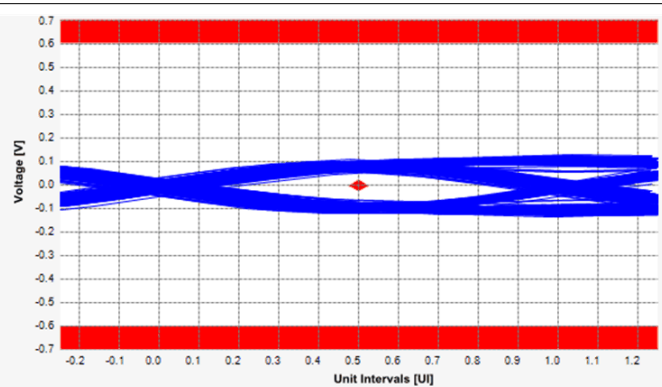
图 7-8. PCIe Gen 3 TX Eye Diagram
