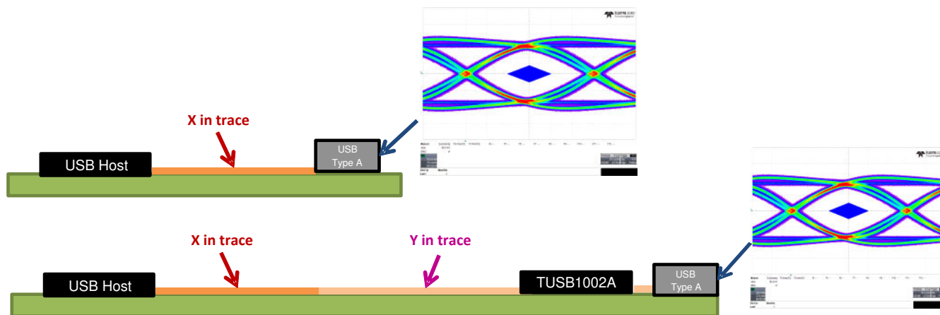
图 6-1. Linear Equalizer
