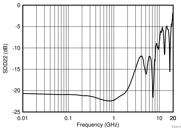
图 5-13. SDD22 Return Loss
