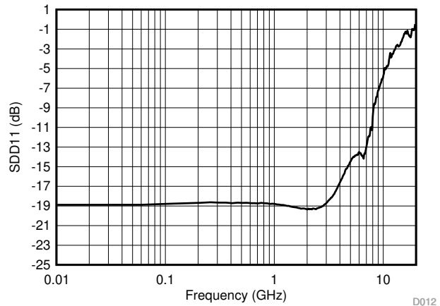
图 5-12. SDD11 Return Loss
