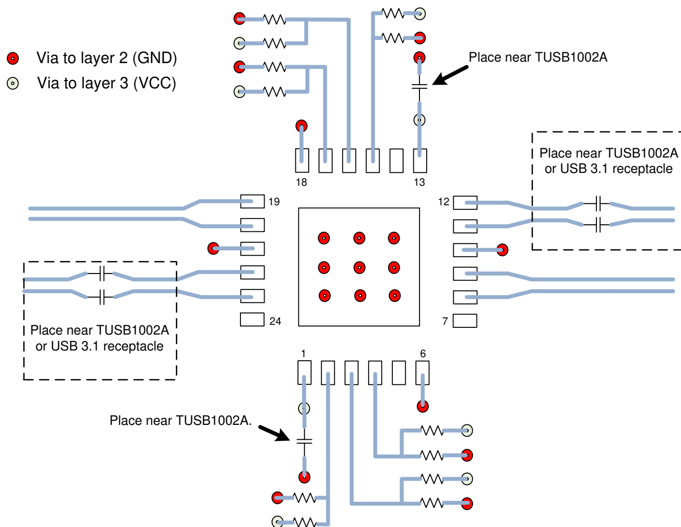
图 7-9. Example Layout
