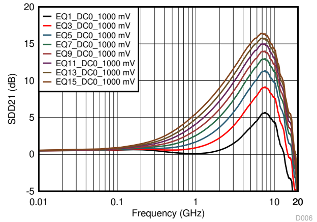
图 5-6. 1000mV DC0 Gain Odd EQ Settings Curves
