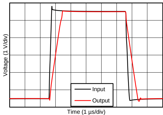
图 25. 过载恢复
