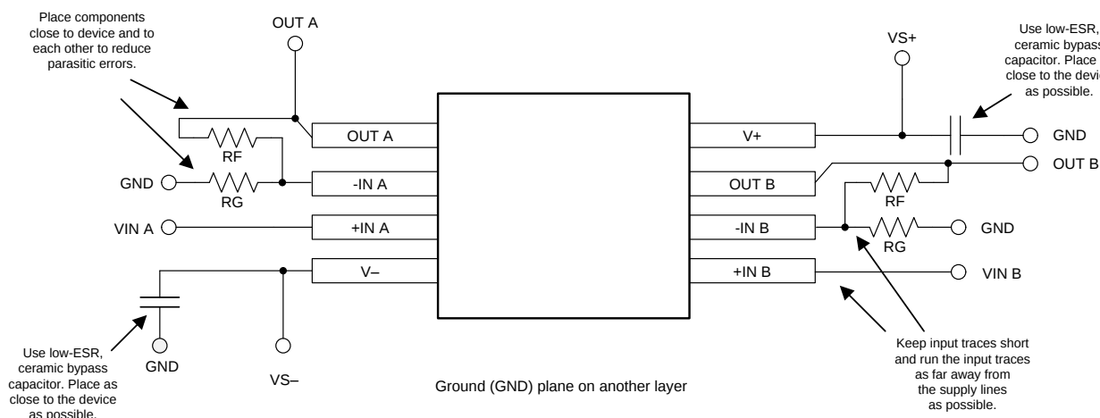
图 39. 布局示例
