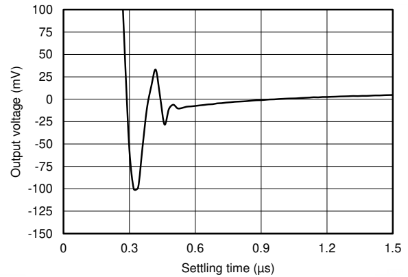
图 7-34. 大信号建立时间 (负)
