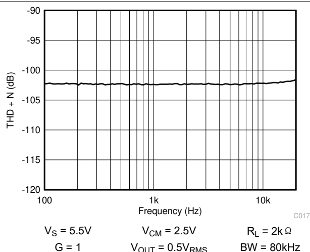
图 7-16. THD+N 与频率间的关系
