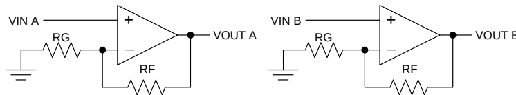
图 38. 图 39 的原理图表示
