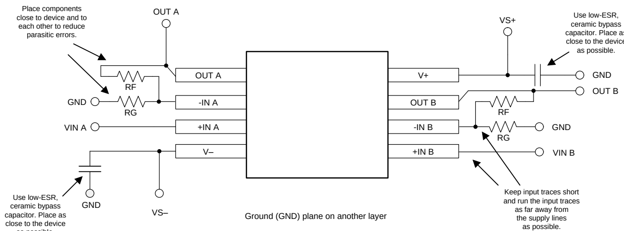
图 39. 布局示例
