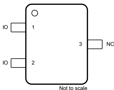
图 4-1. DBZ 封装， 3 引脚 SOT-23 (顶视图)
