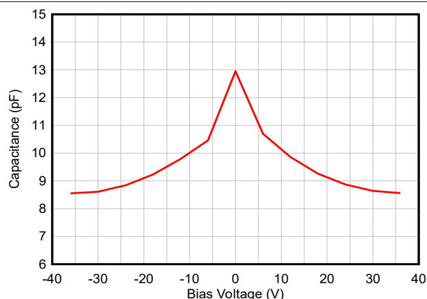
图 5-3. 电容与偏置电压之间的关系
