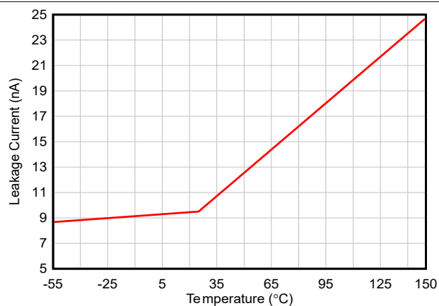
图 5-4. 漏电流与温度间的关系
