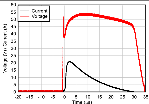
图 5-2. 8/20 \mu s 浪涌响应
