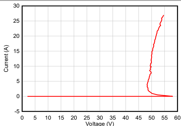
图 5-1. 正 TLP 曲线
