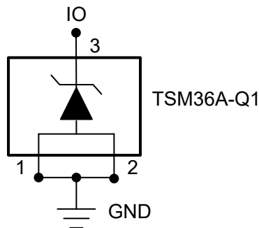
功能方框图
