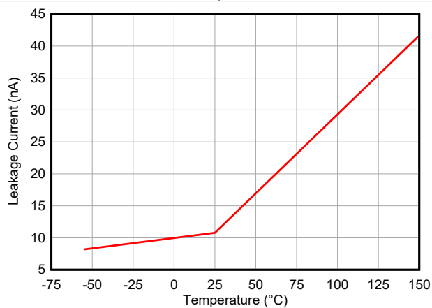
图 6-3. 漏电流与温度之间的关系
