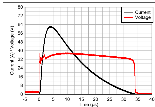
图 6-1. 8/20 \mu s 浪涌响应
