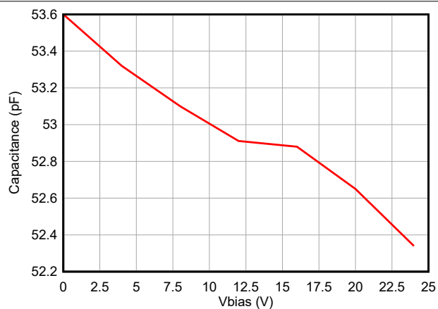
图 6-2. 电容与偏置电压之间的关系
