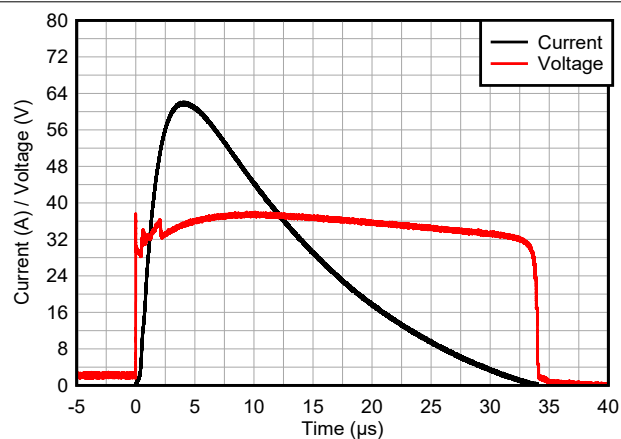
图 6-1. 8/20 \mu s 浪涌响应
