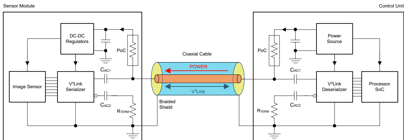
图 7-1. 同轴电缆供电 (PoC) 系统图
