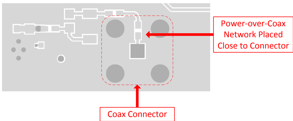
图 7-9. TSER953 同轴电缆供电布局
