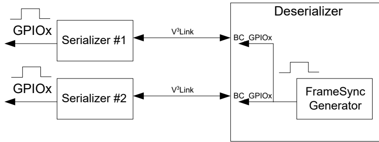
图 6-5. 内部帧同步
