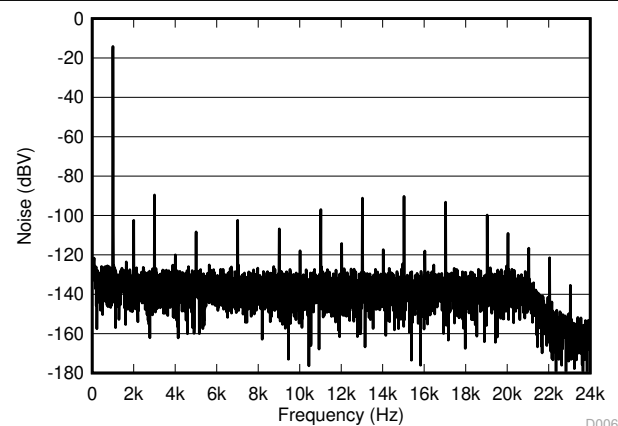
图 5-6. 具有 1W 输出的噪声 FFT
