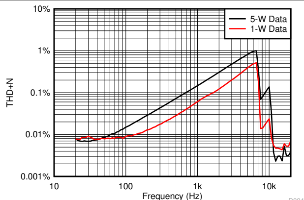
图 5-4. THD+N 与频率间的关系
