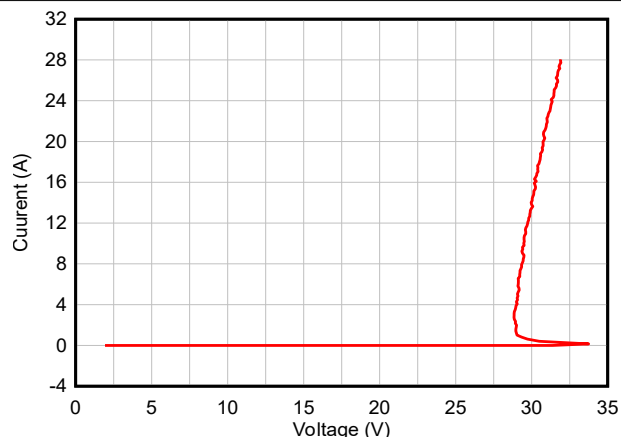
图 5-4. 正 TLP 曲线 - TSD24-Q1
