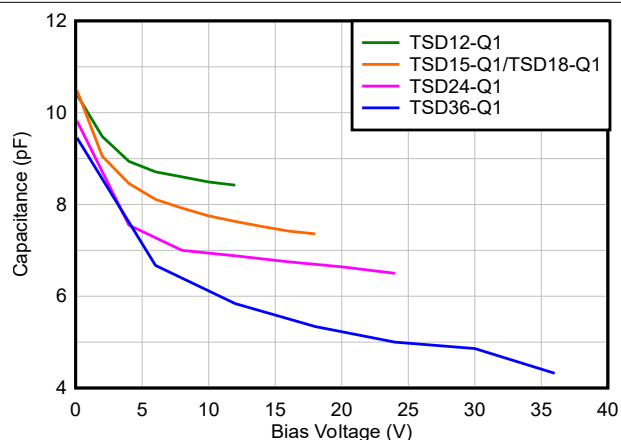
图 5-6. 电容与偏置电压之间的关系
