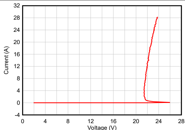
图 5-3. 正 TLP 曲线 - TSD18-Q1
