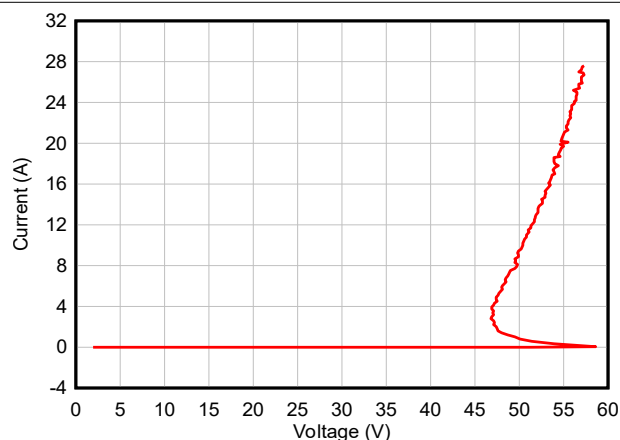
图 5-5. 正 TLP 曲线 - TSD36-Q1
