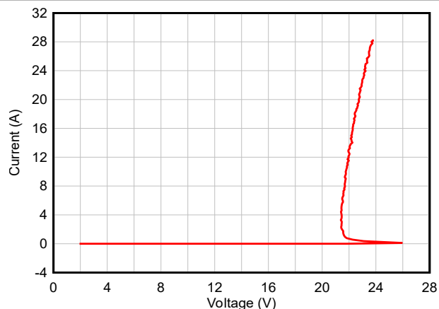
图 5-2. 正 TLP 曲线 - TSD15-Q1
