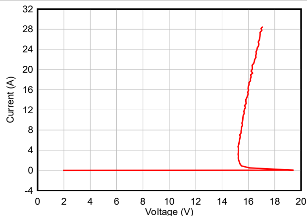
图 5-1. 正 TLP 曲线 - TSD12-Q1
