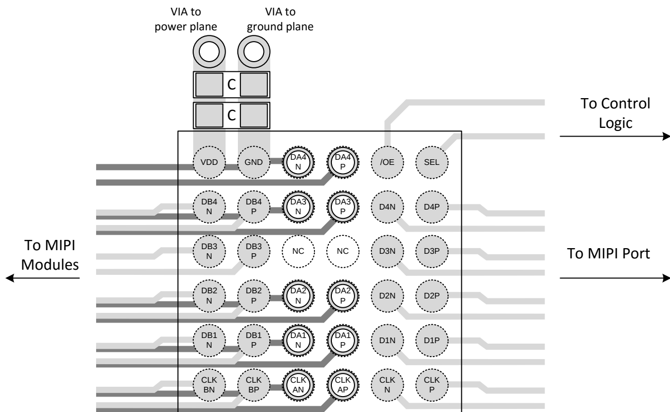
图 26. Layout Example
