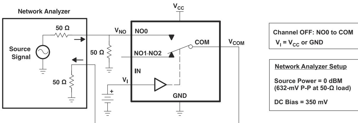
图 7-8. Off Isolation ( O_{iso} )
