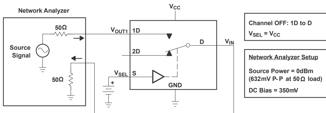
图 6-2. OFF Isolation ( O_{ISO} )
