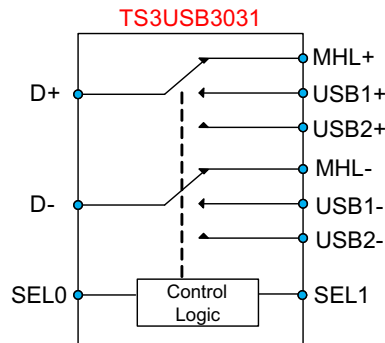
开关图
