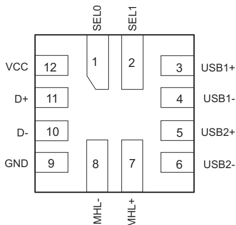
图 4-2. RMG Package, 12-Pin VQFN (Bottom View)
