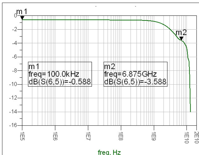
图 5-3. Bandwidth for MHL Switch
