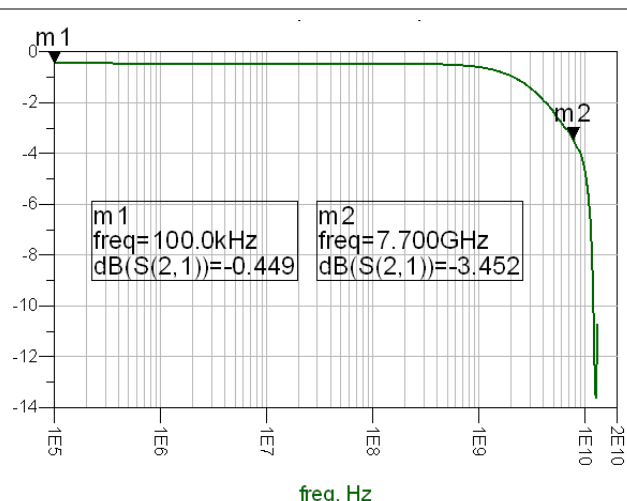
图 5-4. Bandwidth for USB Switch
