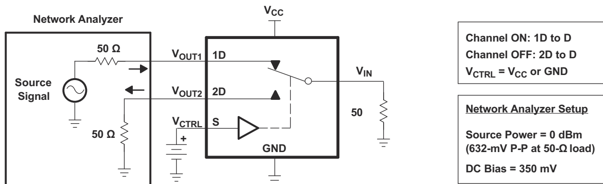
图 6-3. Crosstalk ( X_{TALK} )
