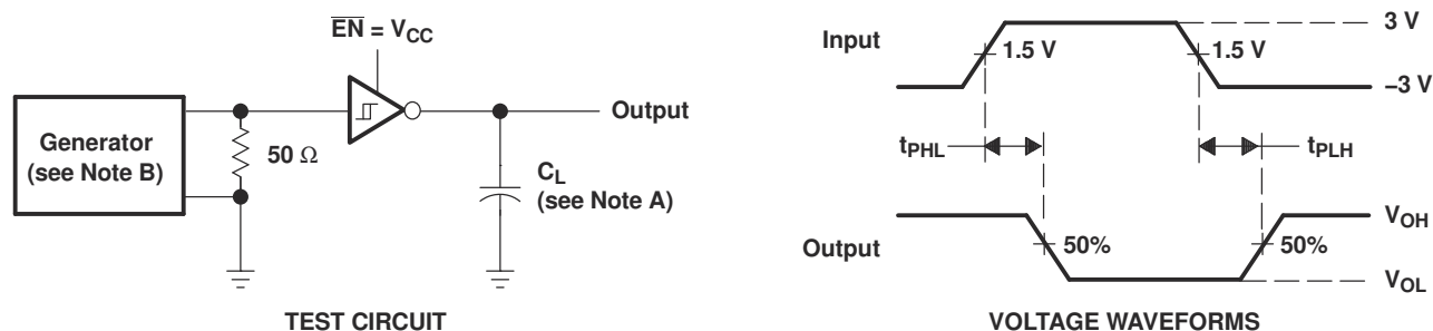
图 6-2. Driver Pulse Skew
