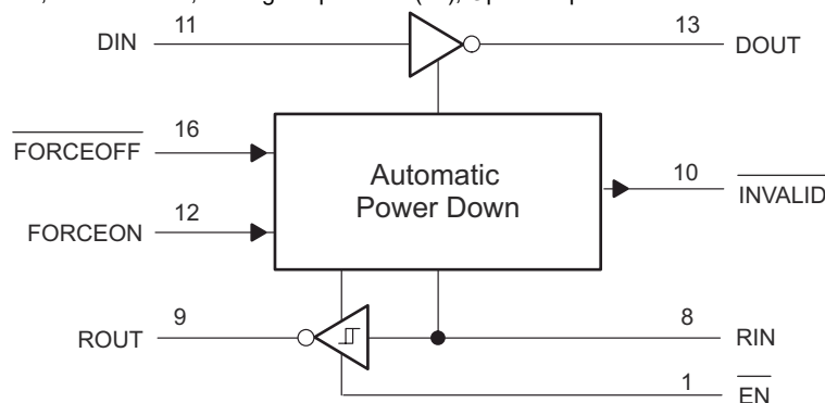
图 7-1. Logic Diagram
