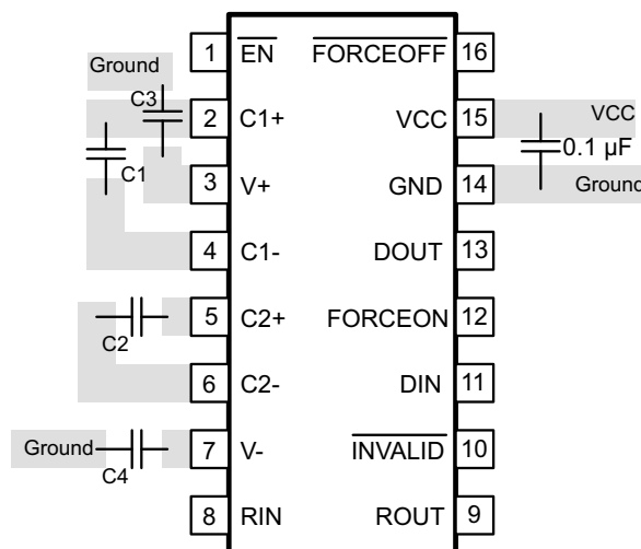
图 8-3. Layout Diagram
