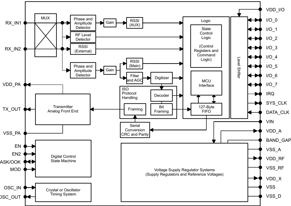
图 1-1. 方框图
