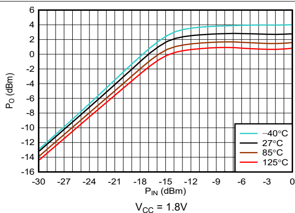
图 5-42. 整个温度范围内输出功率 ( P_O ) 与输入功率 ( P_{IN} ) 间的关系
