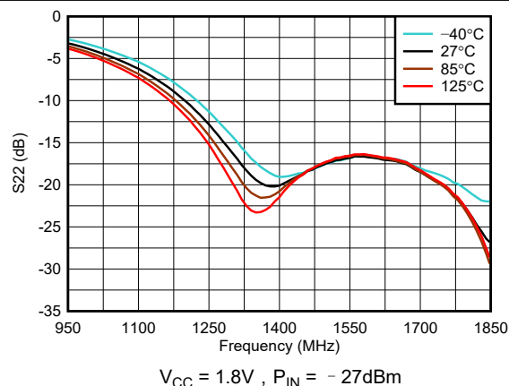
图 5-40. 整个温度范围内的输出回波损耗 (S22)
