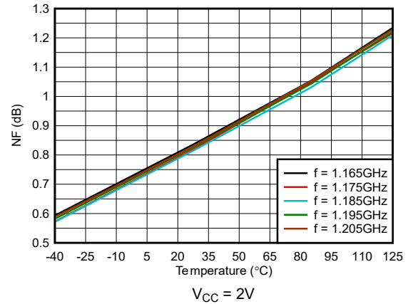
图 5-50. 整个频率范围内 NF 与温度间的关系
