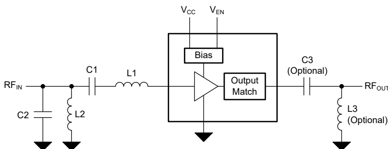
图 6-3. TRF3302 典型多 GNSS 频段配置
