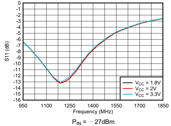
图 5-32. 整个 V_{CC} 内的输入回波损耗 ( S_{11} )
