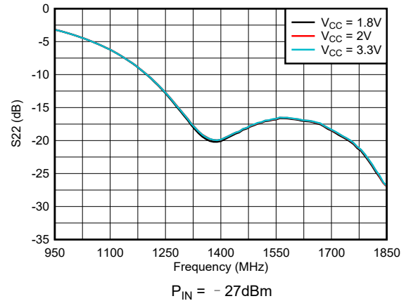
图 5-34. 整个 V_{CC} 内的输出回波损耗 ( S_{22} )
