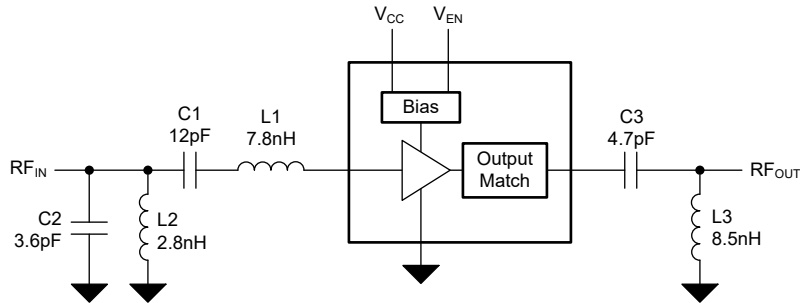
图 7-1. 配置中的 TRF3302 涵盖 L1、L2 和 L5 GPS 频段
