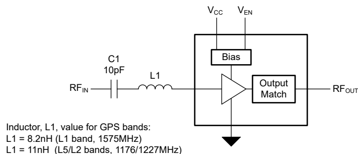
图 6-2. TRF3302 典型单 GNSS 频段配置
