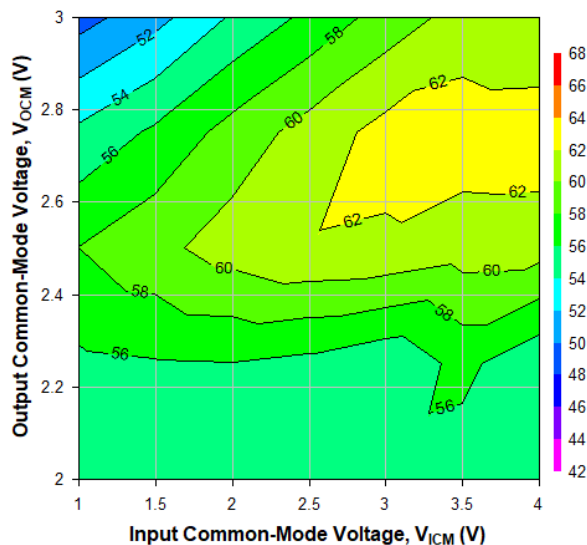
图 6-49. 500MHz 时不同 V_{\text{ICM}} 和 V_{\text{OCM}} 条件下的 OIP2，Ch1
