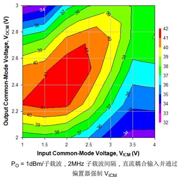
图 6-46. 500MHz 时不同 V_{ICM} 和 V_{OCM} 条件下的 OIP3, Ch2
