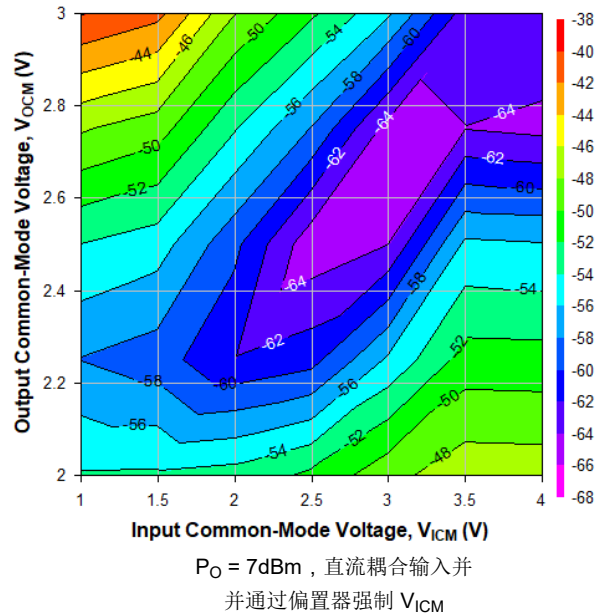
图 6-60. 2GHz 时不同 V_{\text{ICM}} 和 V_{\text{OCM}} 条件下的 HD2, Ch2
