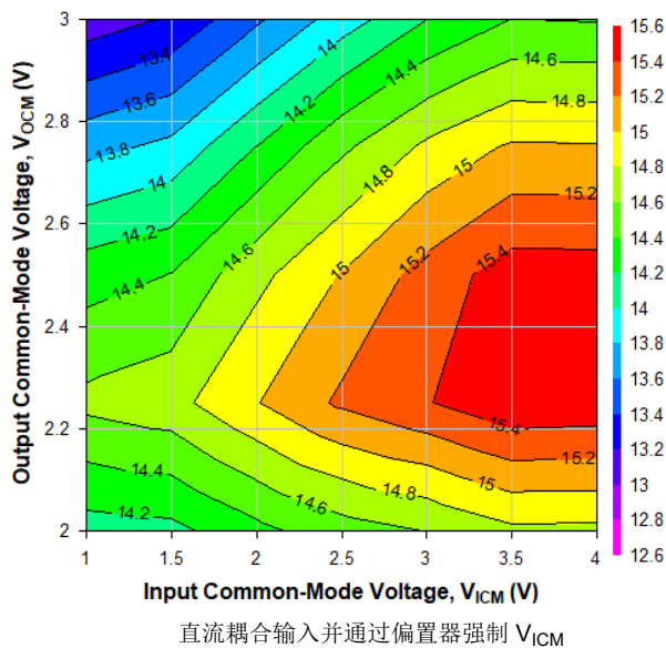
图 6-56. 2GHz 时不同 V_{ICM} 和 V_{OCM} 条件下的 OP1dB, Ch2
