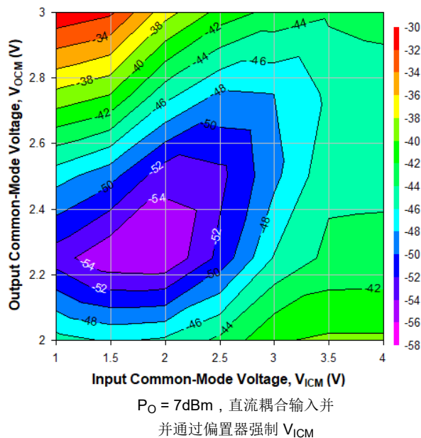
图 6-63. 2GHz 时不同 V_{ICM} 和 V_{OCM} 条件下的 HD3, Ch1
