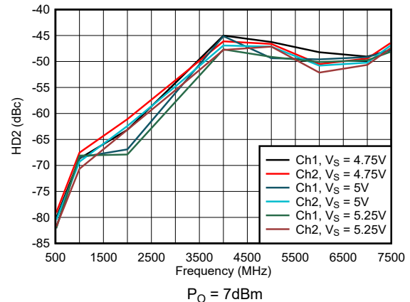
图 6-34. 整个电源电压范围内的 HD2
