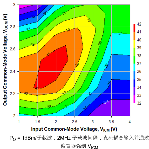
图 6-45. 500MHz 时不同 V_{ICM} 和 V_{OCM} 条件下的 OIP3, Ch1
