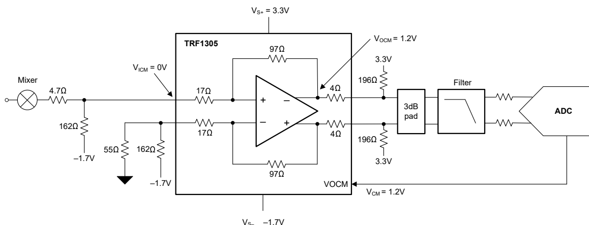
图 8-6. TRF1305C2 用作零中频接收器中的 ADC 驱动器
