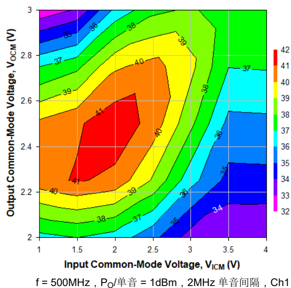
图 8-8. 输入和输出共模电压情况下的 OIP3
