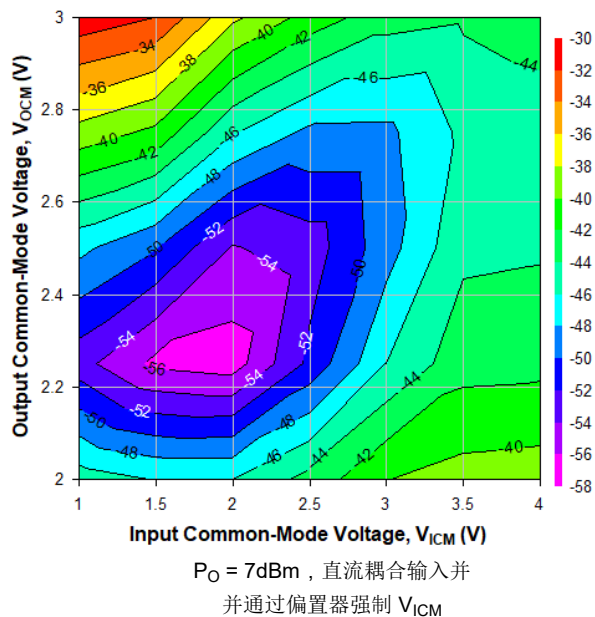
图 6-64. 2GHz 时不同 V_{ICM} 和 V_{OCM} 条件下的 HD3, Ch2
