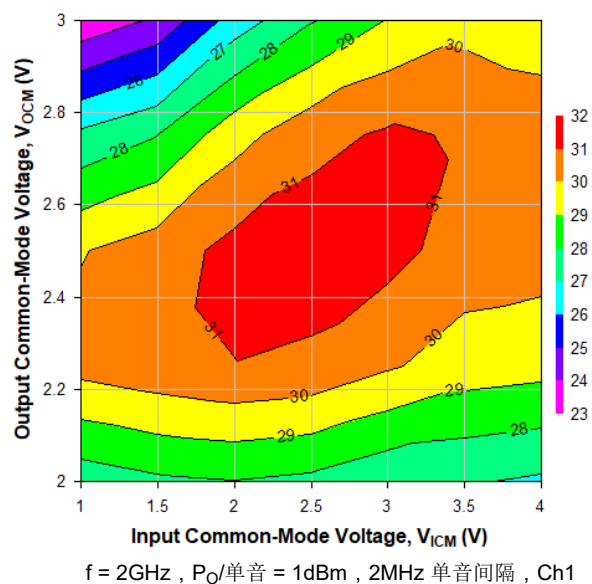
图 8-9. 输入和输出共模电压情况下的 OIP3
