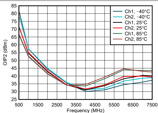
图 6-94. 整个温度范围内的 OIP2
