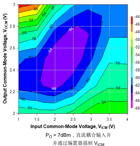
图 6-61. 500MHz 时不同 V_{ICM} 和 V_{OCM} 条件下的 HD3, Ch1
