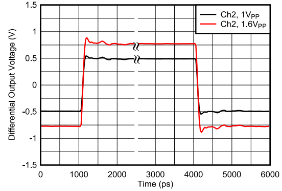
图 6-66. 阶跃响应
