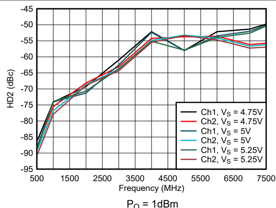
图 6-36. 整个电源电压范围内的 HD2
