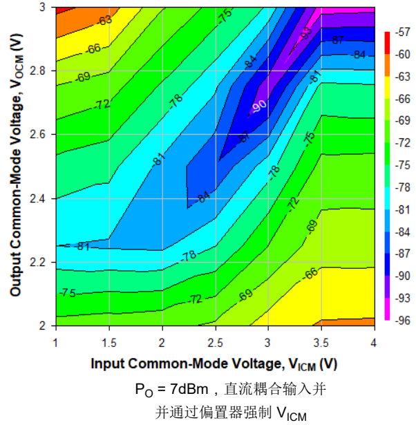
图 6-58. 500MHz 时不同 V_{\text{ICM}} 和 V_{\text{OCM}} 条件下的 HD2, Ch2
