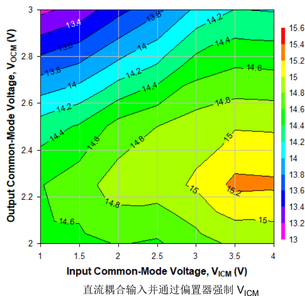
图 6-53. 500MHz 时不同 V_{ICM} 和 V_{OCM} 条件下的 OP1dB, Ch1
