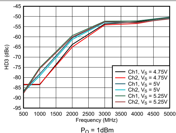
图 6-40. 整个电源电压范围内的 HD3
