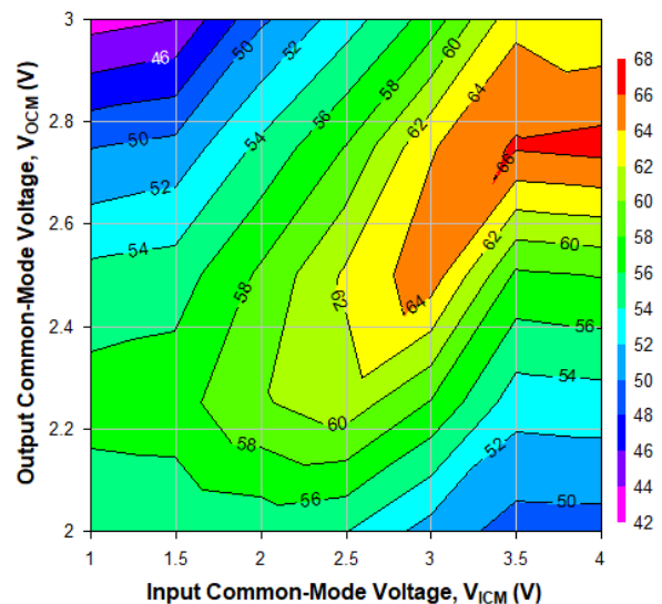
图 6-50. 500MHz 时不同 V_{\text{ICM}} 和 V_{\text{OCM}} 条件下的 OIP2，Ch2
