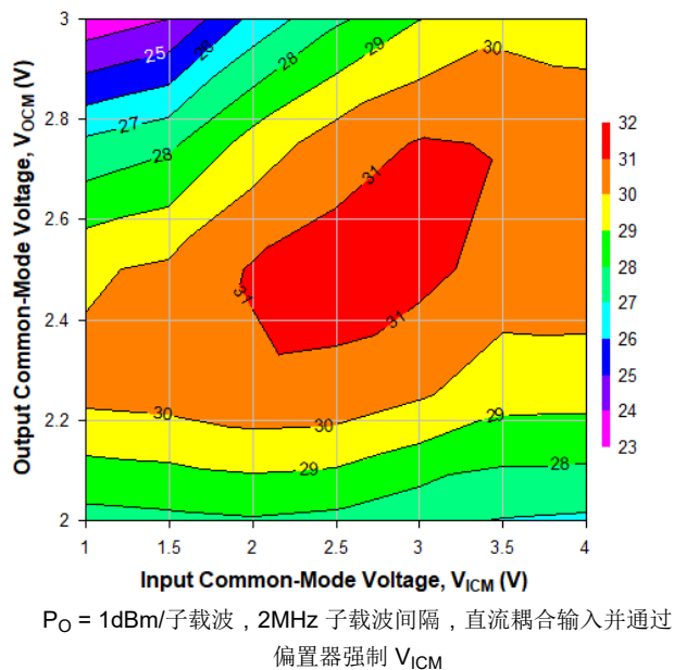
图 6-48. 2GHz 时不同 V_{ICM} 和 V_{OCM} 条件下的 OIP3, Ch2
