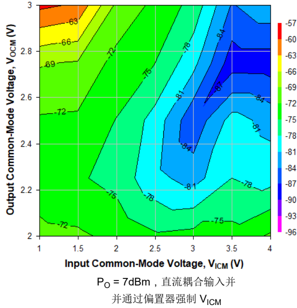
图 6-57. 500MHz 时不同 V_{\text{ICM}} 和 V_{\text{OCM}} 条件下的 HD2, Ch1
