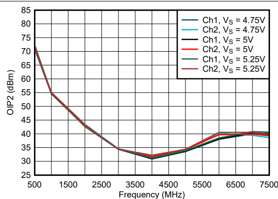
图 6-95. 整个电源电压范围内的 OIP2
