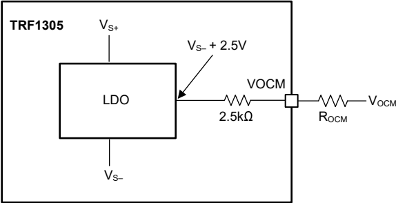
图 7-1. 输出共模控制
