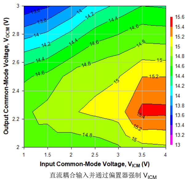
图 6-54. 500MHz 时不同 V_{ICM} 和 V_{OCM} 条件下的 OP1dB, Ch2
