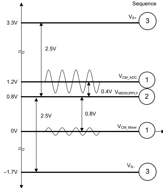
图 8-7. 在给定的共模电压下选择电源电压
