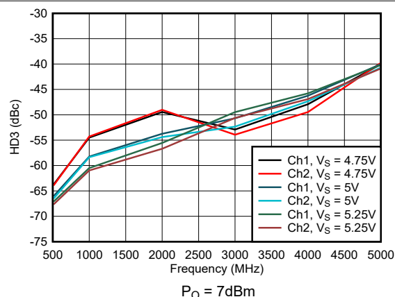
图 6-38. 整个电源电压范围内的 HD3
