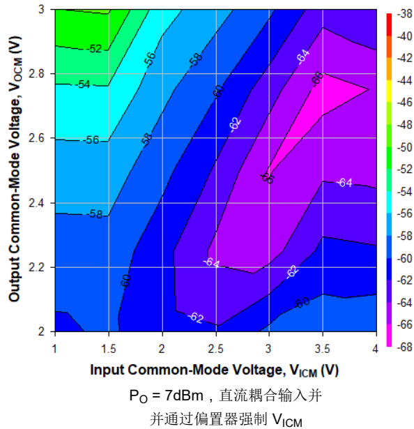
图 6-59. 2GHz 时不同 V_{\text{ICM}} 和 V_{\text{OCM}} 条件下的 HD2, Ch1
