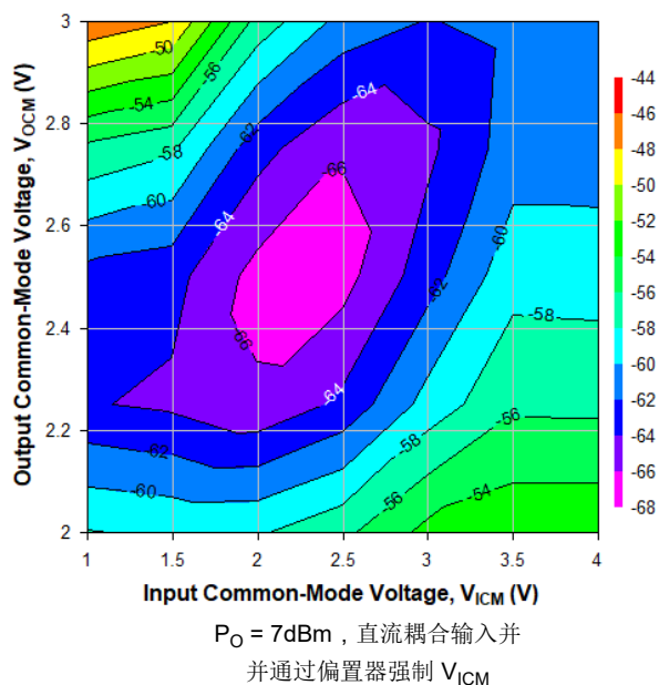
图 6-62. 500MHz 时不同 V_{ICM} 和 V_{OCM} 条件下的 HD3, Ch2
