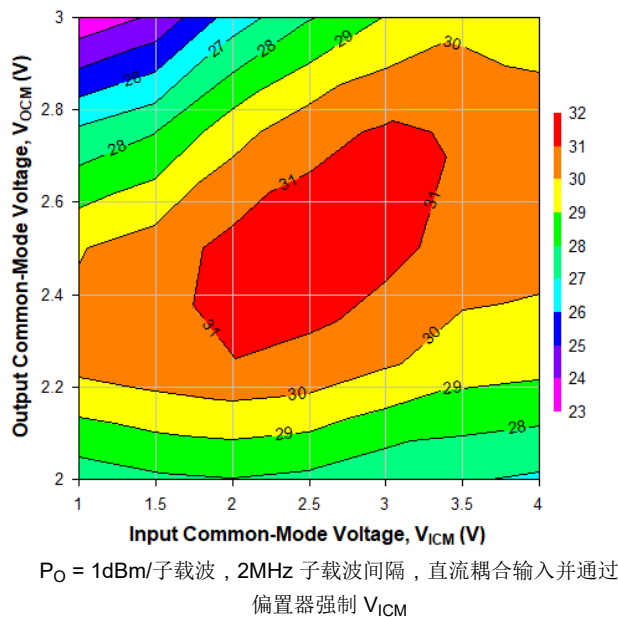
图 6-47. 2GHz 时不同 V_{ICM} 和 V_{OCM} 条件下的 OIP3, Ch1
