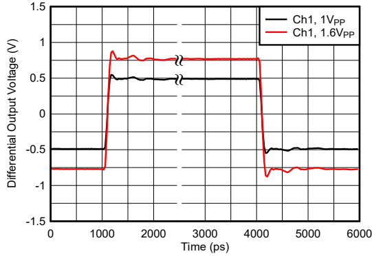
图 6-65. 阶跃响应
