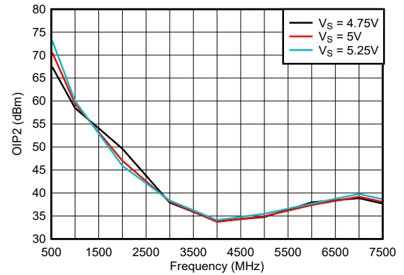
图 6-72. 整个电源电压范围内的 OIP2
