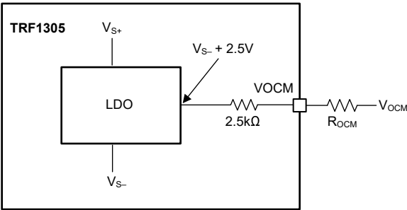
图 7-1. 输出共模控制
