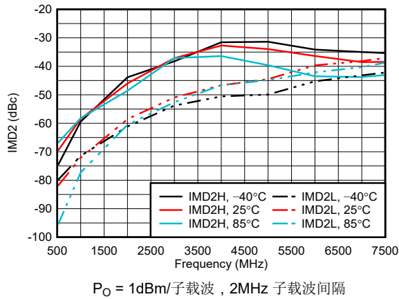
图 6-75. 整个温度范围内的 IMD2
