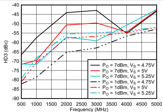
图 6-82. 整个输出功率和电源电压范围内的 HD3
