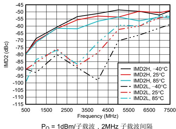
图 6-25. 整个温度范围内的 IMD2
