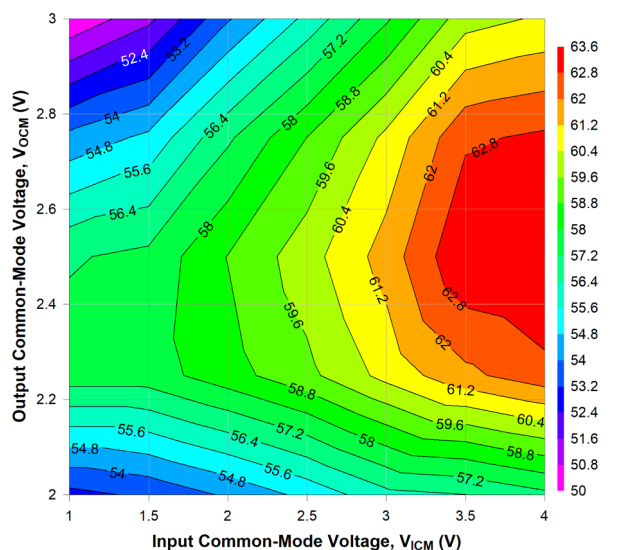
P_O = 1\text{dBm}/\text{子载波} , 2MHz 子载波间隔, 直流耦合输入并通过偏置器强制 V_{ICM}
