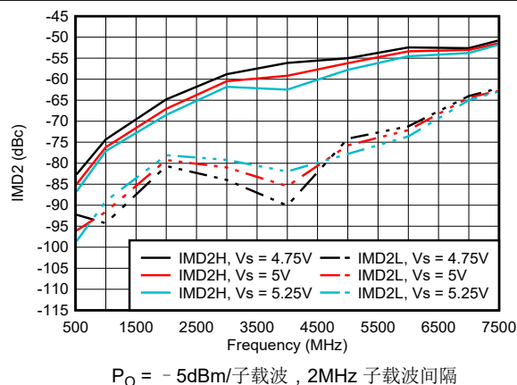
图 6-28. 整个电源电压范围内的 IMD2
