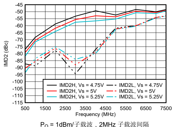
图 6-26. 整个电源电压范围内的 IMD2
