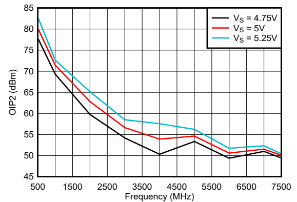
图 6-22. 整个电源电压范围内的 OIP2
