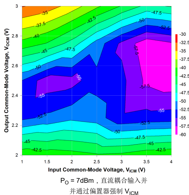
图 6-46. 2GHz 时不同 V_{\text{ICM}} 和 V_{\text{OCM}} 条件下的 HD3
