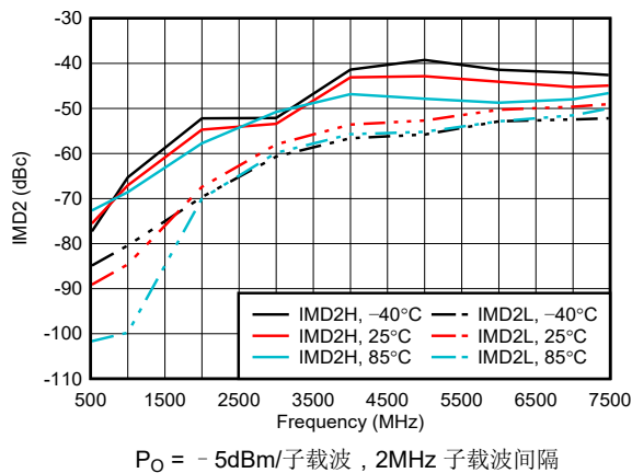
图 6-77. 整个温度范围内的 IMD2
