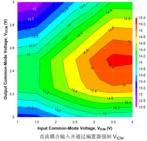
图 6-42. 2GHz 时不同 V_{ICM} 和 V_{OCM} 条件下的 OP1dB
