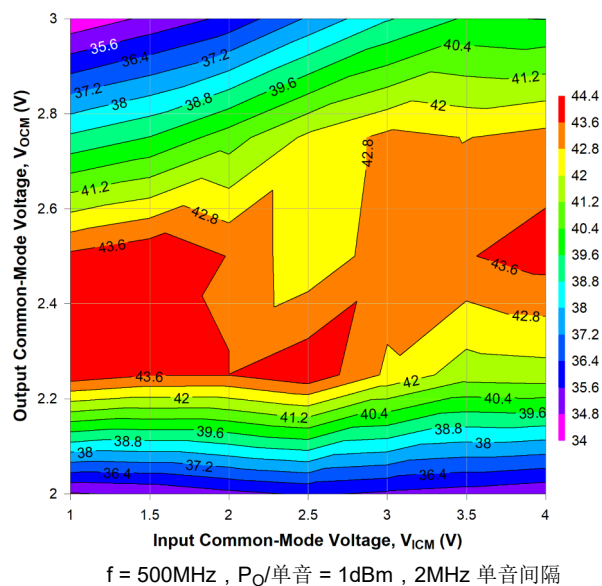
图 8-8. 输入和输出共模电压情况下的 OIP3
