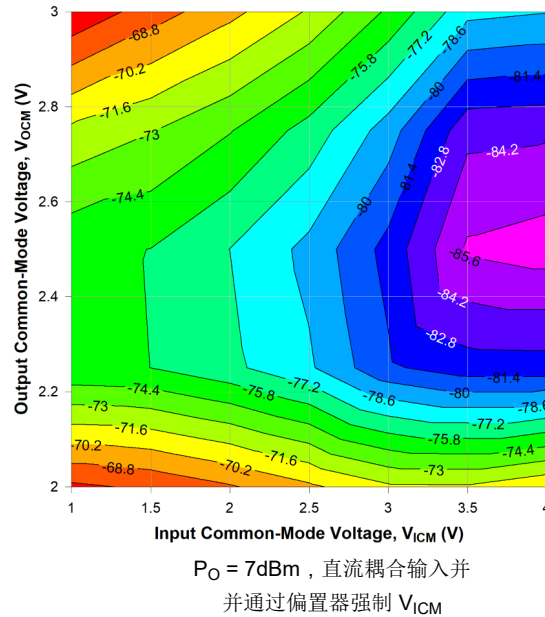
图 6-43. 500MHz 时不同 V_{ICM} 和 V_{OCM} 条件下的 HD2
