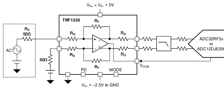
驱动高速 ADC、采用 S2D 配置的 TRF1305C1
