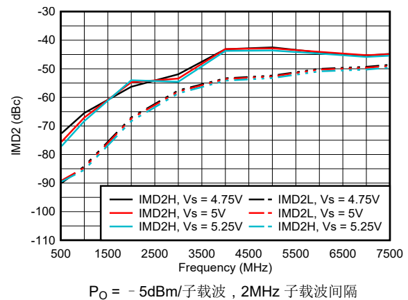
图 6-78. 整个电源电压范围内的 IMD2
