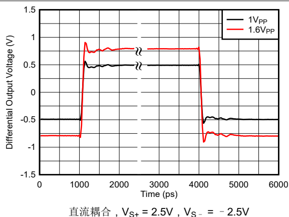
图 6-47. 阶跃响应
