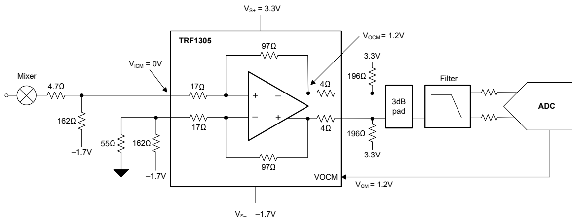
图 8-6. TRF1305C1 用作零中频接收器中的 ADC 驱动器
