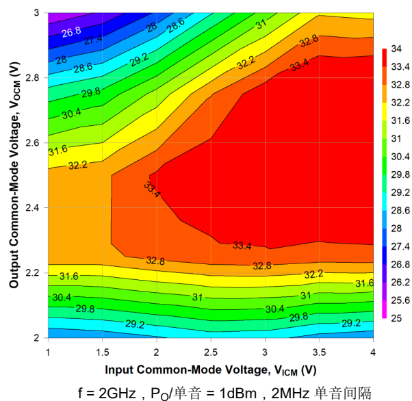
图 8-9. 输入和输出共模电压情况下的 OIP3
