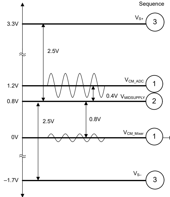
图 8-7. 在给定的共模电压下选择电源电压
