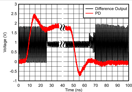
图 6-88. 上电和断电时序
