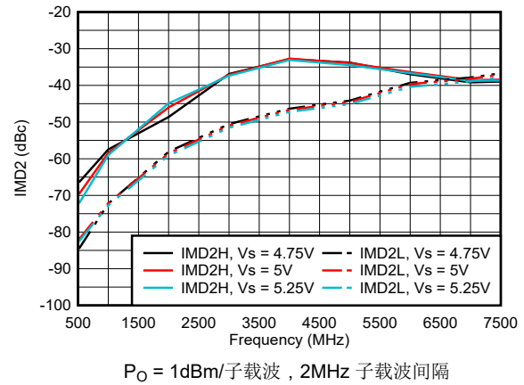
图 6-76. 整个电源电压范围内的 IMD2
