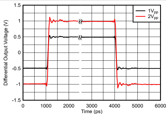
图 6-87. 阶跃响应
