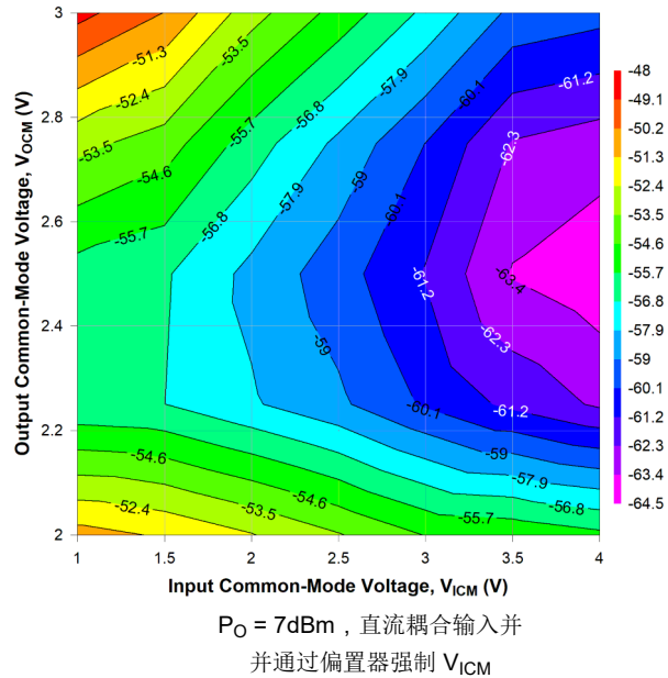
图 6-44. 2GHz 时不同 V_{ICM} 和 V_{OCM} 条件下的 HD2
