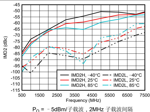
图 6-27. 整个温度范围内的 IMD2
