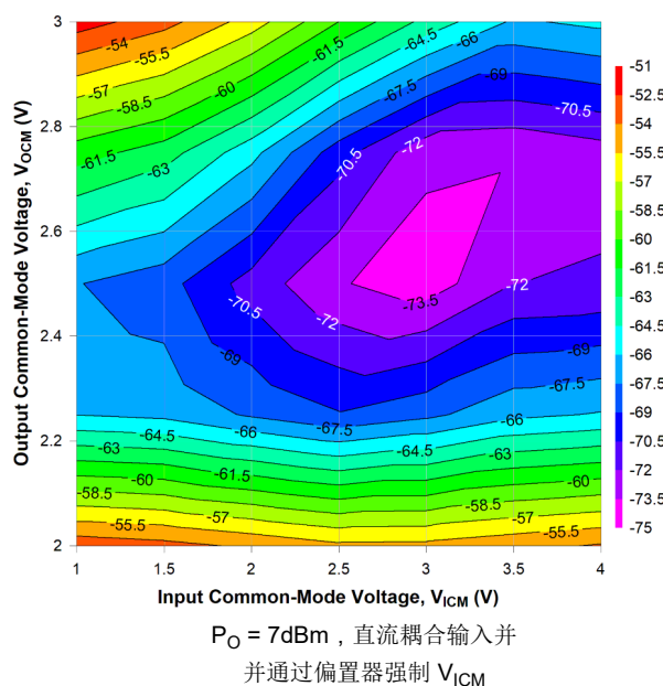
图 6-45. 500MHz 时不同 V_{\text{ICM}} 和 V_{\text{OCM}} 条件下的 HD3
