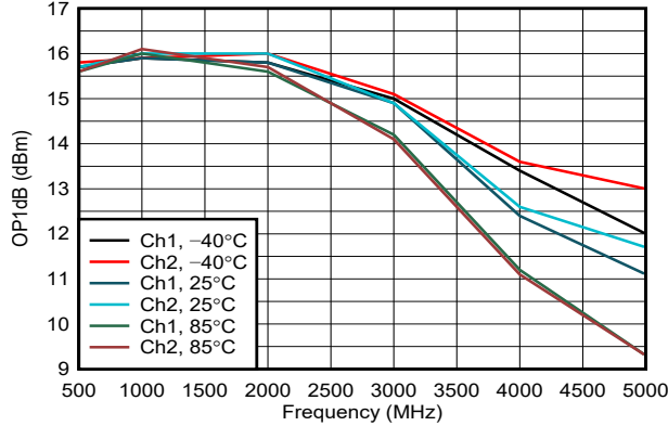
图 6-19. 整个温度范围内的 OP1dB
