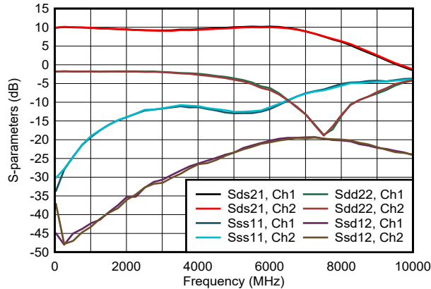
图 6-25. S2D 配置中的 S 参数
