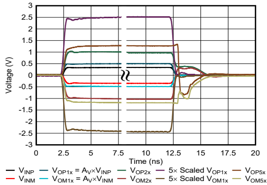
图 6-31. 阶跃响应
