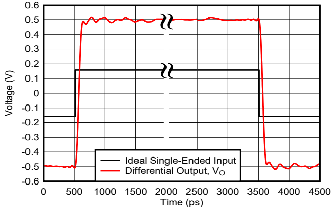
图 6-31. 阶跃响应
