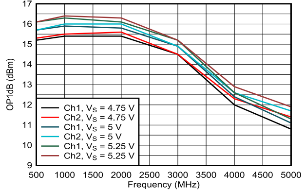
图 6-20. 整个电源电压范围内的 OP1dB
