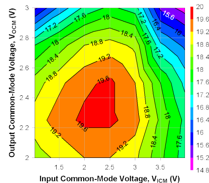
图 6-16. 2GHz 时不同 V_{\text{ICM}} 和 V_{\text{OCM}} 条件下的 OIP3
