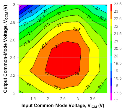
图 6-15. 500MHz 时不同 V_{\text{ICM}} 和 V_{\text{OCM}} 下的 OIP3
