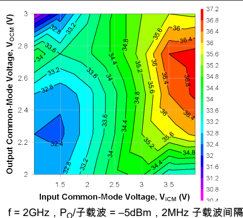
图 8-9. 输入和输出共模电压情况下的 OIP3
