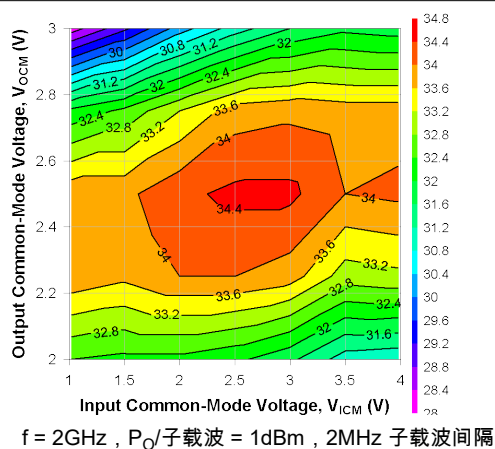
图 8-8. 输入和输出共模电压情况下的 OIP3
