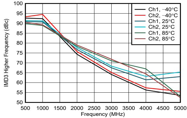
图 6-13. 整个温度范围内的 IMD3 更高
