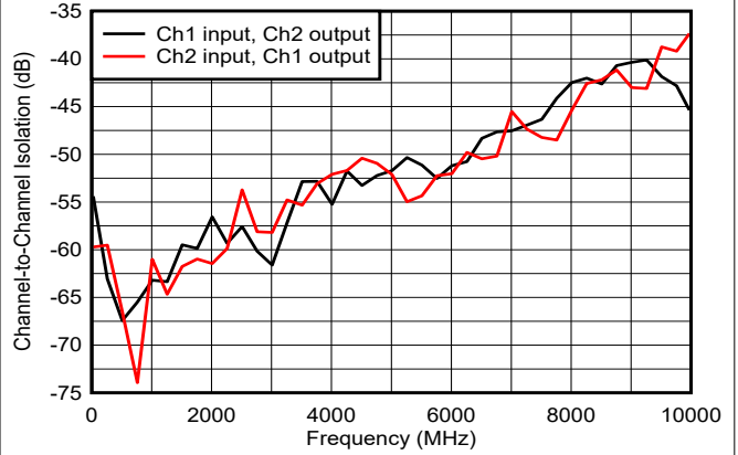
图 6-32. 通道间隔离
