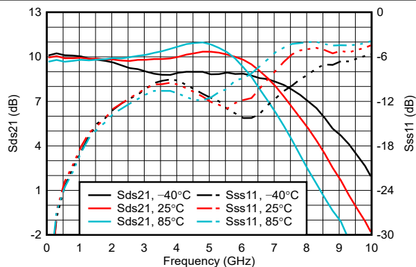
S2D, 具有 50\ \Omega 源阻抗时每个输入引脚上的 P_{\text{IN}} = -20\text{dBm} , 剥离至 INP 和 OUTP/OUTM 引脚
