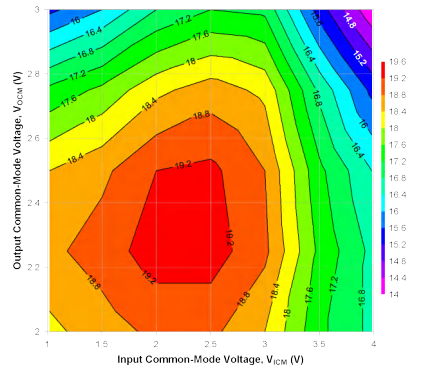
P_O = 1\text{dBm}/\text{子载波} , 2MHz 子载波间隔, 直流耦合输入并通过偏置器强制 V_{ICM} 图 6-18. 5GHz 时不同 V_{ICM} 和 V_{OCM} 条件下的 OIP3
