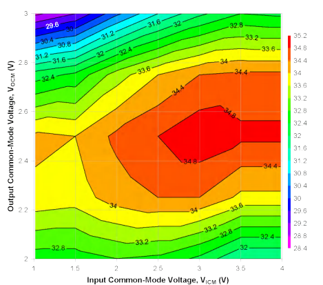
图 8-8. 输入和输出共模电压情况下的 OIP3
