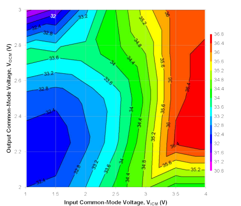
图 8-9. 输入和输出共模电压情况下的 OIP3
