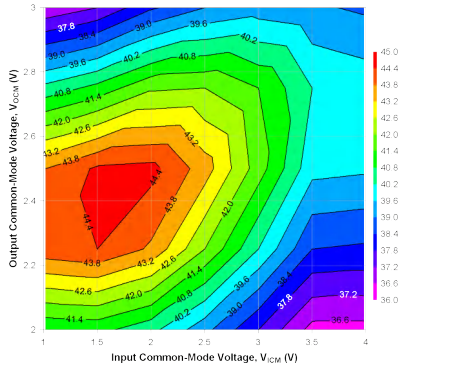
P_O = 1\text{dBm}/\text{子载波} , 2MHz 子载波间隔, 直流耦合输入并通过偏置器强制 V_{ICM} 图 6-15. 500MHz 时不同 V_{ICM} 和 V_{OCM} 条件下的 OIP3
