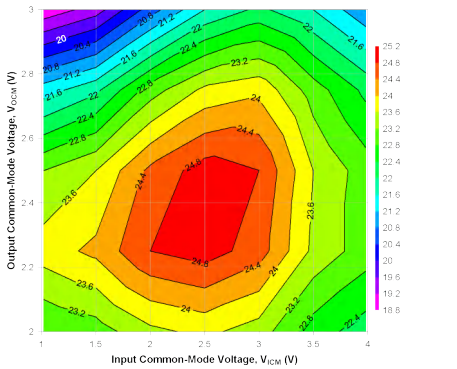
P_O = 1\text{dBm}/\text{子载波} , 2MHz 子载波间隔, 直流耦合输入并通过偏置器强制 V_{ICM} 图 6-17. 4GHz 时不同 V_{ICM} 和 V_{OCM} 条件下的 OIP3
