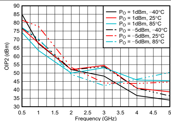
S2D, 所示为每个子载波的 P_O , 2MHz 子载波间隔, 剥离至 INP 和 OUTP/OUTM 引脚
