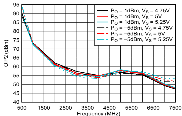
图 6-20. 整个电源电压范围内的 OIP2
