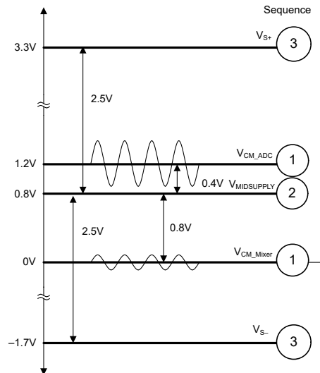
图 8-7. 在给定的共模电压下选择电源电压
