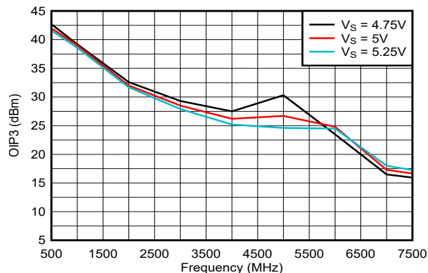
图 6-8. 整个电源电压范围内的 OIP3
