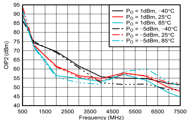
图 6-19. 整个温度范围内的 OIP2
