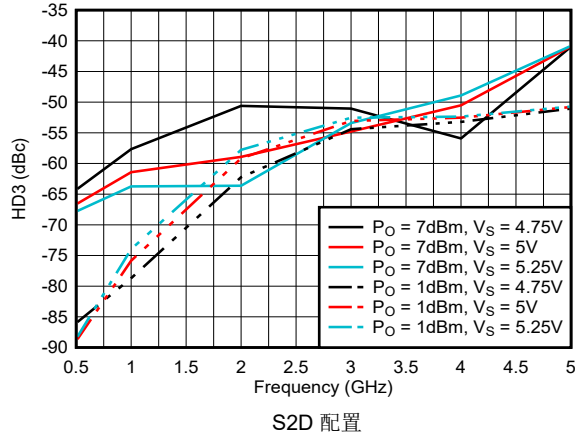
图 6-37. 整个电源电压和输出功率范围内的 HD3
