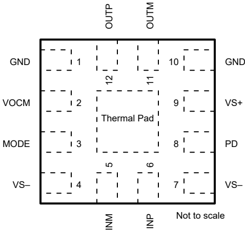
图 5-1. RPV 封装，12 引脚 WQFN-FCRLF ( 顶视图 )
