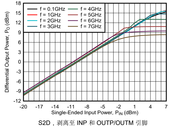
图 6-40. 单端输入与差分输出功率间的关系
