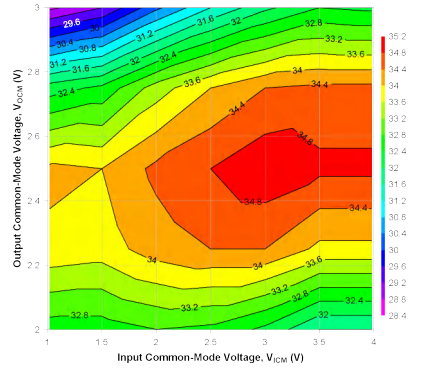
P_O = 1\text{dBm}/\text{子载波} , 2MHz 子载波间隔, 直流耦合输入并通过偏置器强制 V_{ICM} 图 6-16. 2GHz 时不同 V_{ICM} 和 V_{OCM} 条件下的 OIP3
