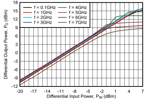
图 6-26. 差分输入与差分输出功率间的关系
