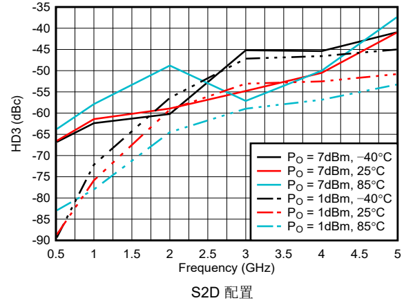
图 6-38. 整个温度和输出功率范围内的 HD3
