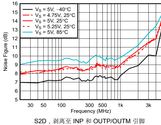
图 6-41. S2D 配置中的噪声系数
