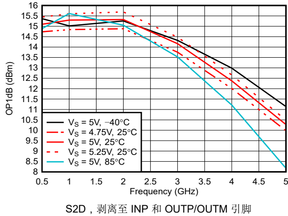
图 6-39. 整个电源电压和温度范围内的 OP1dB
