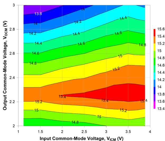
图 6-41. 500MHz 时不同 V_{\text{ICM}} 和 V_{\text{OCM}} 条件下的 OP1dB
