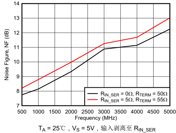
图 8-4. 噪声系数 (NF) 随 R_{IN\_SER} 、 R_{TERM} 的变化
