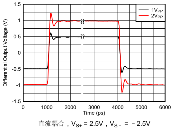
图 6-47. 阶跃响应
