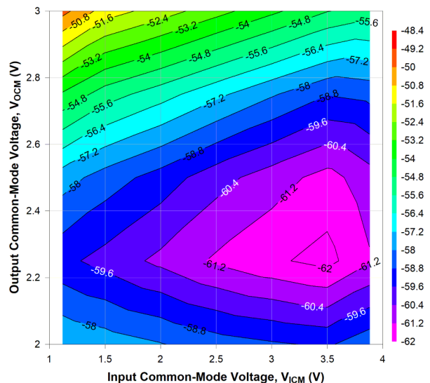
图 6-42. 2GHz 时不同 V_{\text{ICM}} 和 V_{\text{OCM}} 条件下的 OP1dB
