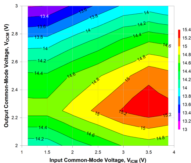
图 6-42. 2GHz 时不同 V_{\text{ICM}} 和 V_{\text{OCM}} 条件下的 OP1dB
