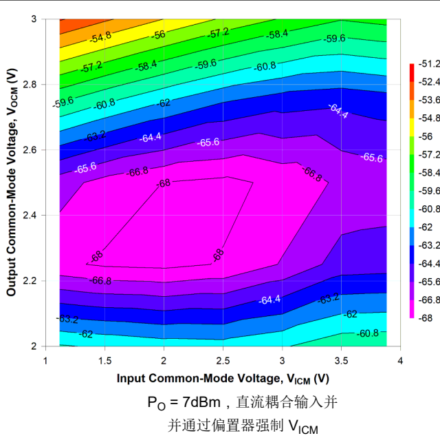
图 6-45. 500MHz 时不同 V_{\text{ICM}} 和 V_{\text{OCM}} 条件下的 HD3
