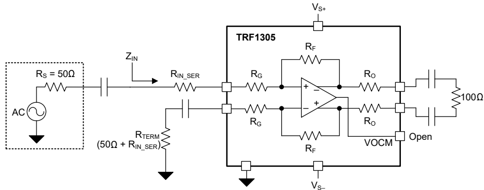
图 8-5. 与 50 Ω 源匹配的交流耦合单端输入
