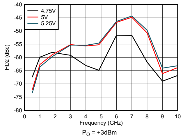
图 5-22. 整个 V_{DD} 范围内的 HD2
