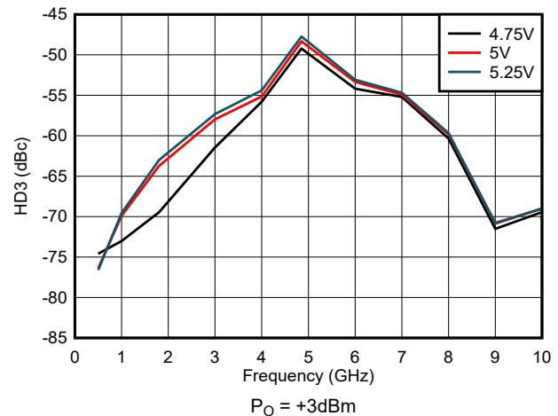
图 5-24. 整个 V_{DD} 范围内的 HD3
