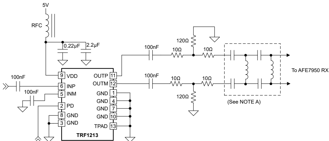
图 7-2. 与 AFE7950 RX 连接
