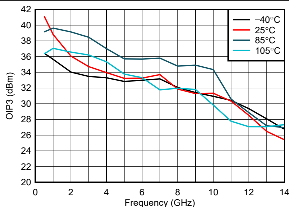
图 5-7. 整个温度范围内的 OIP3
