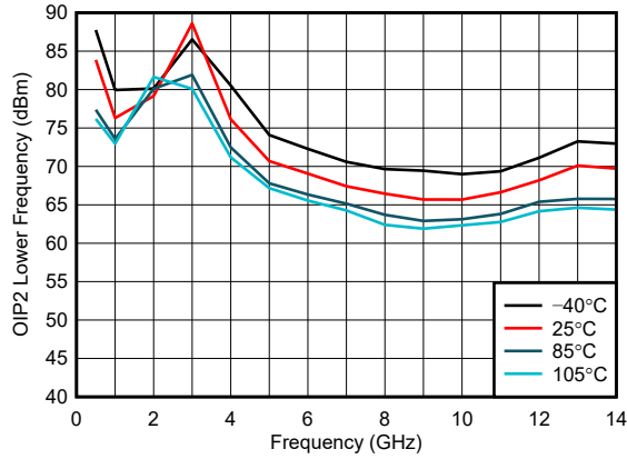
图 5-13. 整个温度范围内的 OIP2 更低
