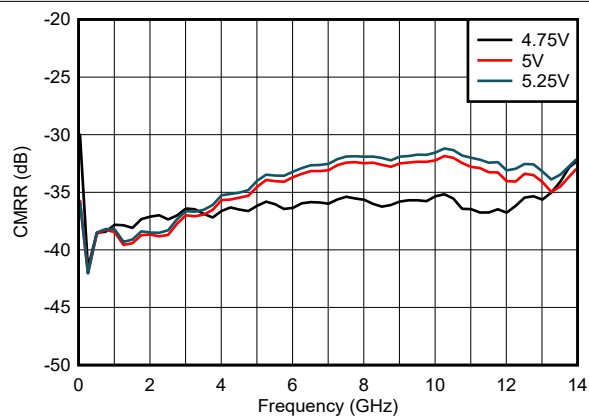
图 5-32. 整个 V_{DD} 范围内的 CMRR
