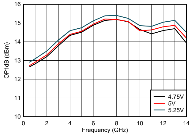
图 5-26. 整个 V_{DD} 范围内的输出 P1dB
