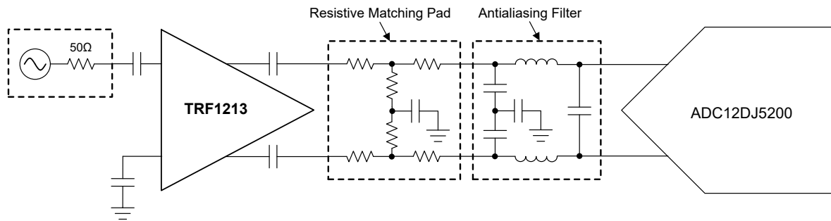
图 7-1. 连接 ADC12DJ5200RF
