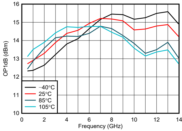
图 5-25. 整个温度范围内的输出 P1dB
