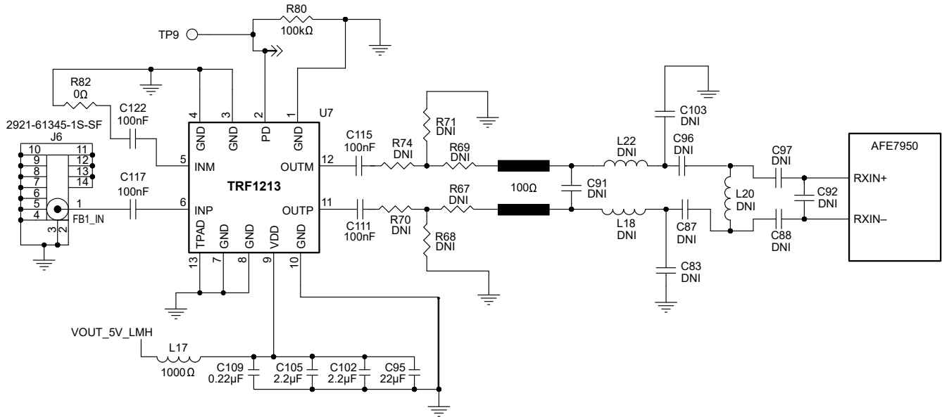
图 7-4. TRF1213 在采用 AFE7950 的接收链中
