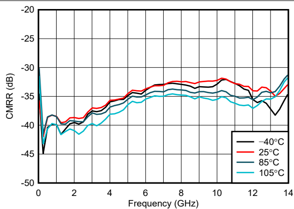
图 5-31. 整个温度范围内的 CMRR
