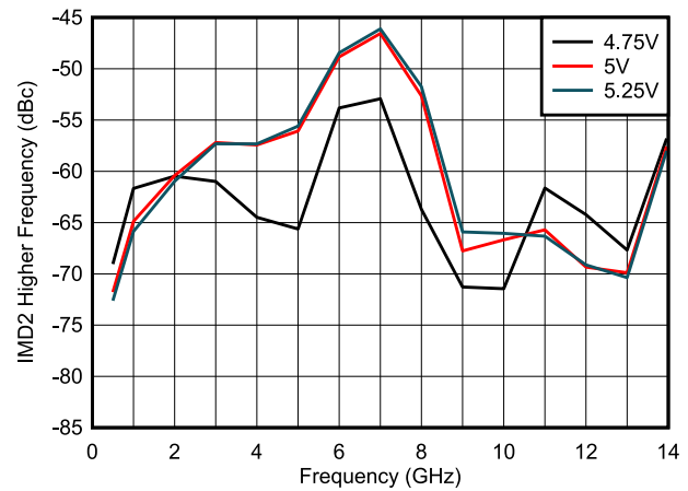
图 5-20. 整个 V_{DD} 范围内的 IMD2 更高
