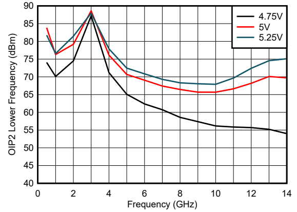
图 5-14. 整个 V_{DD} 范围内的 OIP2 更低
