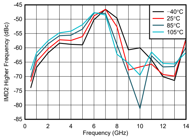
图 5-19. 整个温度范围内的 IMD2 更高
