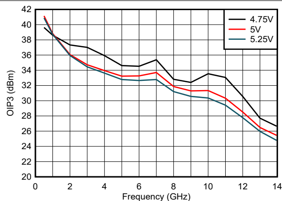
图 5-8. 整个 V_{DD} 范围内的 OIP3
