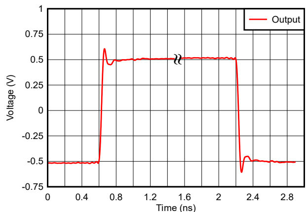
图 5-51. 过载恢复
