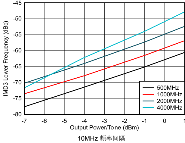
图 5-19. 整个输出功率范围内的 IMD3 较低
