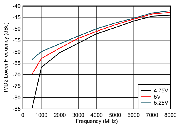
图 5-26. 整个电源电压范围内的 IMD2 更低
