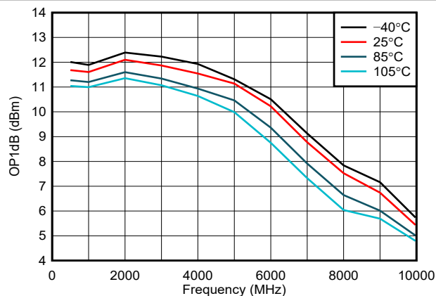
图 5-37. 整个温度范围内的 OP1dB
