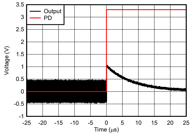
图 5-48. 关断时间
