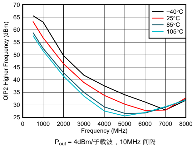
图 5-23. 整个温度范围内的 OIP2 更高
