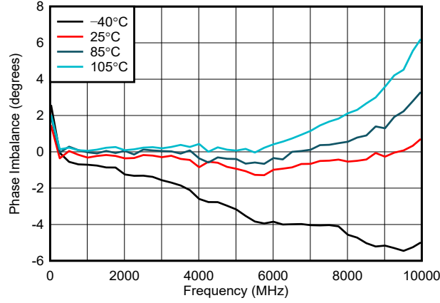
图 5-43. 整个温度范围内的相位不平衡
