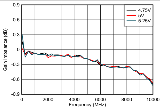
图 5-42. 整个电源电压范围内的增益不平衡
