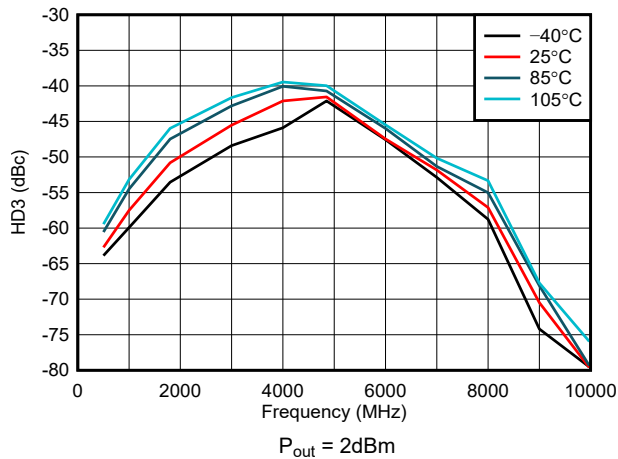
图 5-33. 整个温度范围内的 HD3
