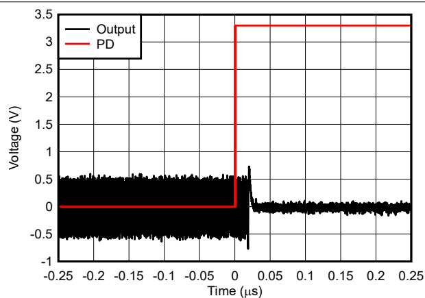
图 5-50. 关断时间
