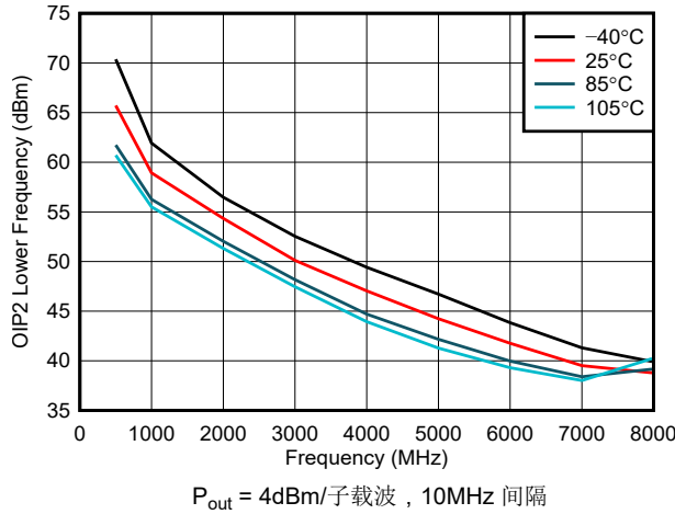
图 5-21. 整个温度范围内的 OIP2 更低
