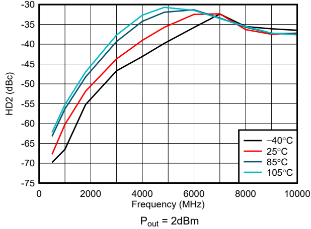
图 5-31. 整个温度范围内的 HD2
