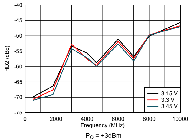
图 5-22. 整个 V_{DD} 范围内的 HD2
