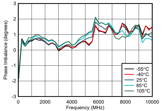
图 5-32. 相位不平衡
