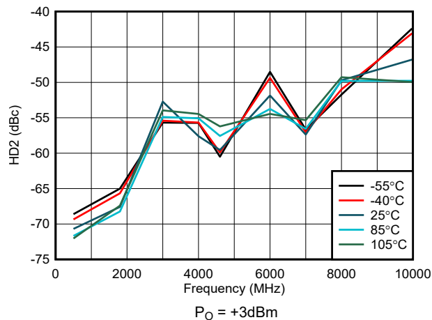
图 5-21. 整个温度范围内的 HD2
