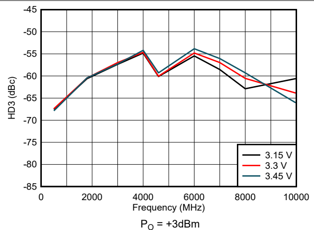
图 5-24. 整个 V_{DD} 范围内的 HD3
