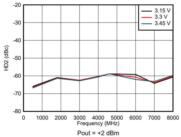
图 6-16. HD2 Across VDD
