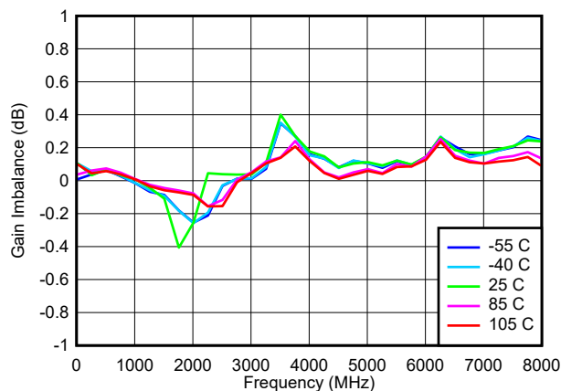
图 6-25. Gain Imbalance
