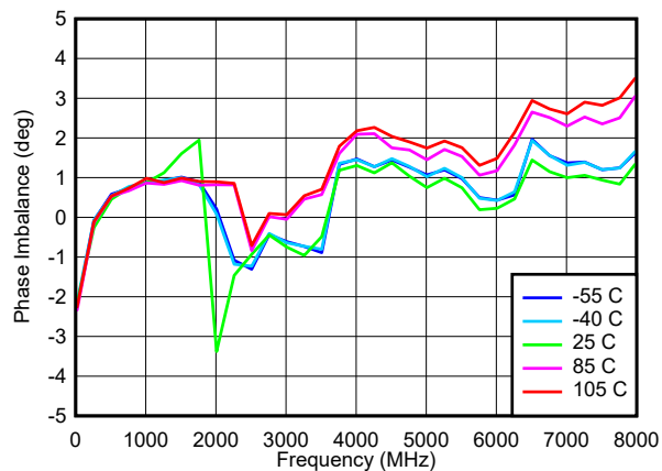
图 6-26. Phase Imbalance
