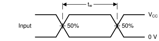
图 6-2. 电压波形，脉冲持续时间
