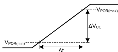
图 7-3. 已知上电状态的电源 ( V_{CC} ) 斜坡特性
