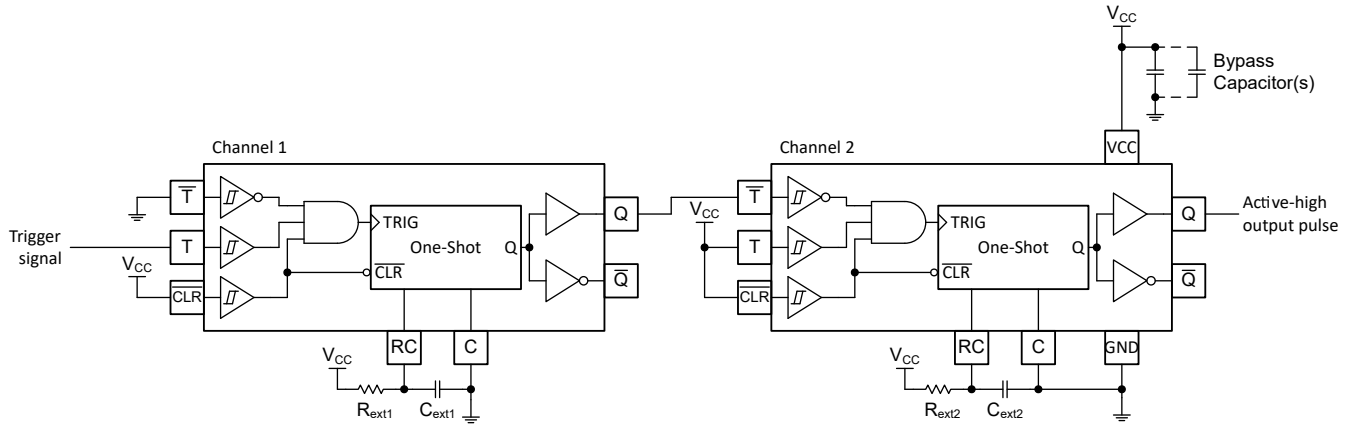
图 8-4. 使用 TPUL2T323 的延迟脉冲发生原理图
