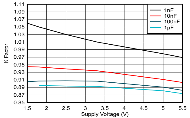
图 5-3. K 系数与电源电压间的关系, R_{ext} = 10\text{k}\Omega
