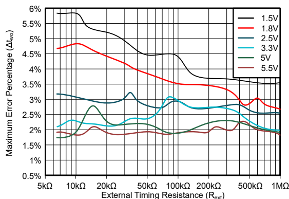
图 5-20. C_{\text{ext}} = 1\text{nF} 时最大输出脉冲宽度误差 (绝对值) 与时序电阻器值间的关系
