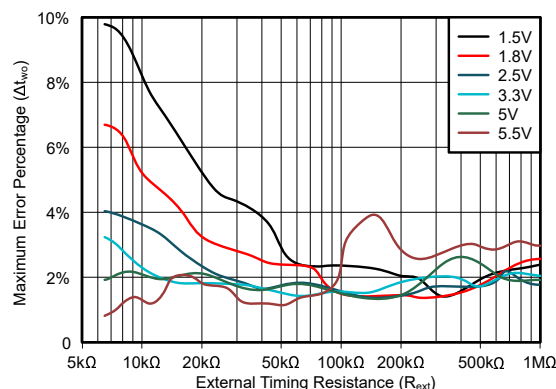
图 5-19. C_{\text{ext}} = 100\text{pF} 时最大输出脉冲宽度误差 (绝对值) 与时序电阻器值间的关系
