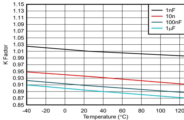
图 5-2. K 系数与温度间的关系, R_{ext} = 10\text{k}\Omega
