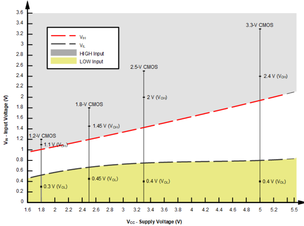
图 7-4. TPULxT 输入电压电平
