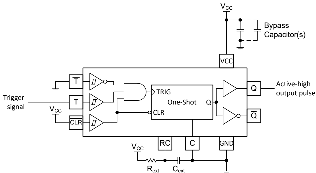
图 8-1. 使用 TPUL2T323 的脉冲发生器原理图
