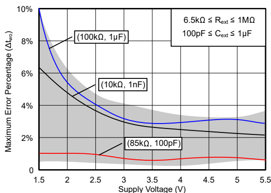
图 5-18. 电源电压范围内的最大输出脉冲宽度误差 (绝对值)
