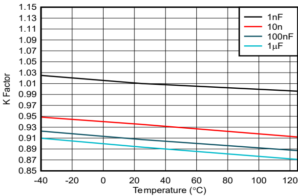
图 5-2. K 系数与温度间的关系， R_{\text{ext}} = 10\text{k}\Omega
