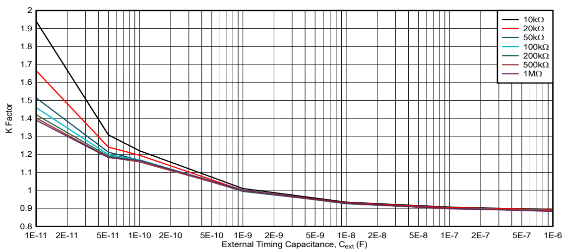
图 5-11. K 系数, V_{CC} = 3.3V , R_{ext} = 10k\Omega 至 1M\Omega
