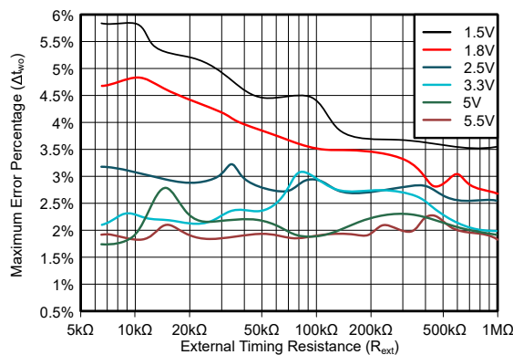
图 5-21. C_{ext} = 1\text{nF} 时最大输出脉冲宽度误差 (绝对值) 与时序电阻器值间的关系
