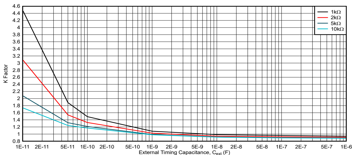
图 5-12. K 系数, V_{CC} = 5V , R_{ext} = 1k\Omega 至 10k\Omega
