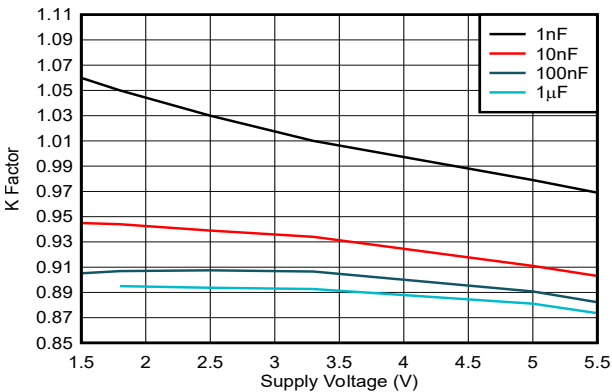
图 5-3. K 系数与电源电压间的关系， R_{\text{ext}} = 10\text{k}\Omega
